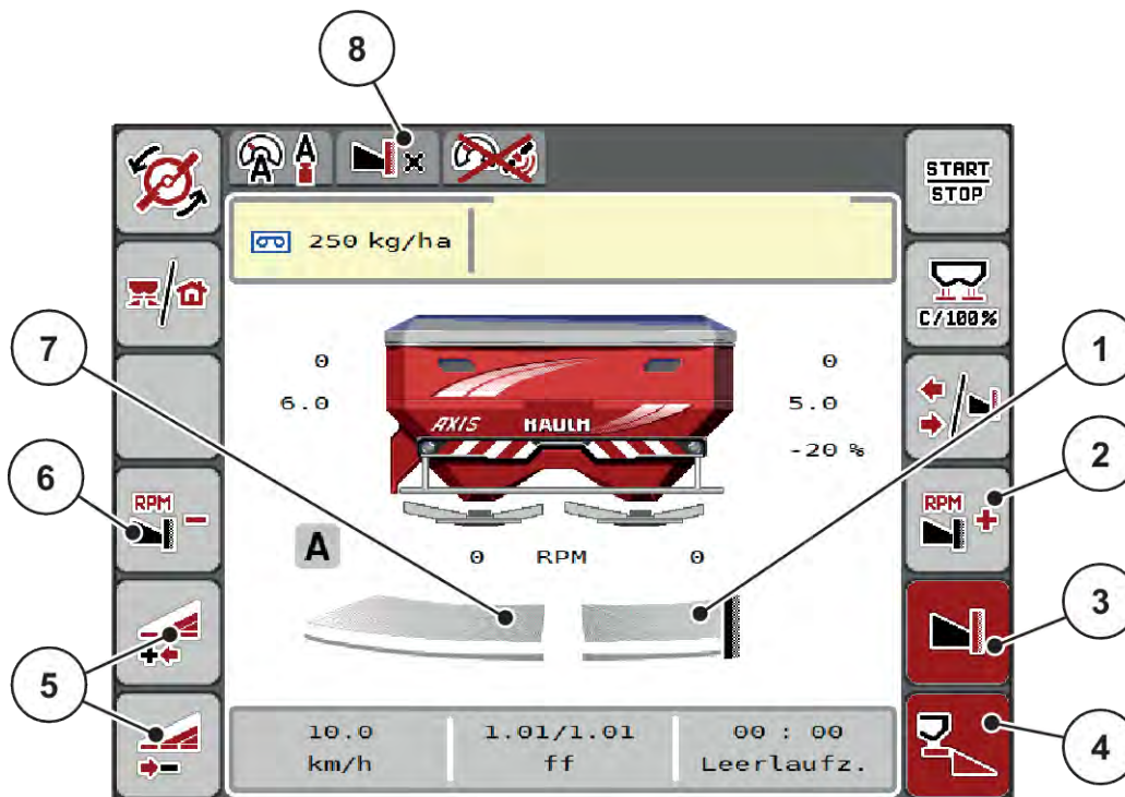
図 43: 左側がセクション散布、右側が境界散布の場合の操作画面
