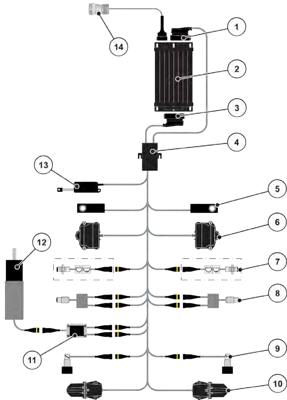
図 6: AXIS-H EMC : 接続図
