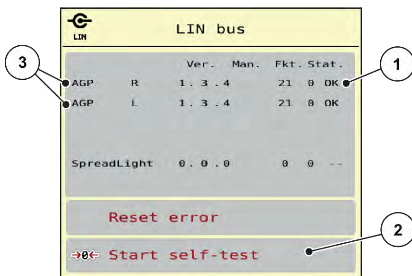
図 25: システム/テスト、例: テスト/診断
