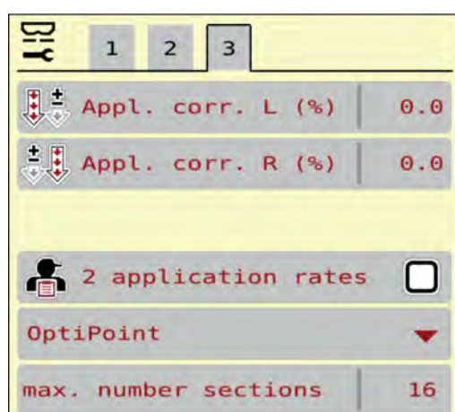
図 20: メニュー 機械設定、タブ3
