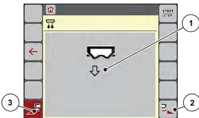
Σχ. 21: Μενού Ταχεία εκκένωση
