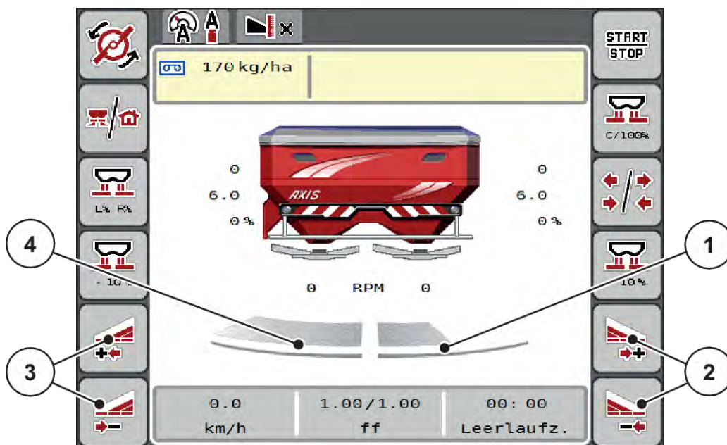
Σχ. 39: Οθόνη λειτουργίας: Τμηματικά εύρη με 4 βαθμίδες
