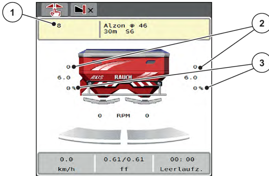
Σχ. 46: Οθόνη λειτουργίας «Κλίμακα MAN»
