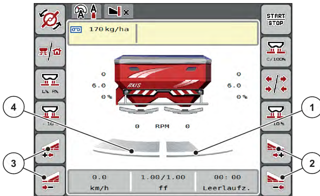
Σχ. 41: Οθόνη λειτουργίας: Αδιαβάθμητη ρύθμιση τμηματικού εύρους
