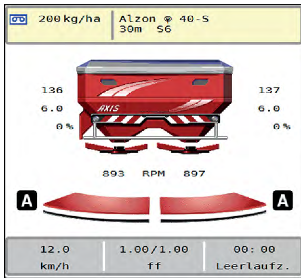
Σχ. 47: Ένδειξη λειτουργίας διασκορπισμού με GPS-Control στην οθόνη λειτουργίας
