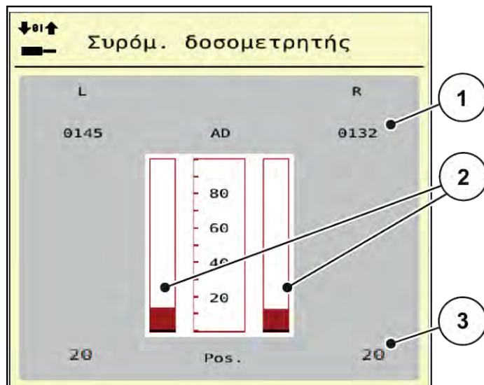
Σχ. 24: Δοκιμή/Διάγνωση, Παράδειγμα: Συρόμ. δοσομετρητής
