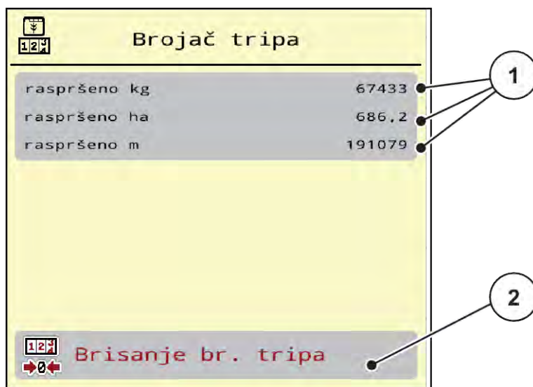
Sl. 26: Izbornik Brojač tripa
