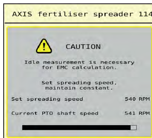
Kuva 48: Tyhjäkäyntimittauksen hälytysnäyttö
