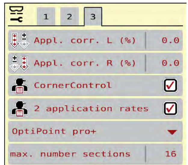
Kuva 26: Valikko Koneasetukset, välilehti 3
