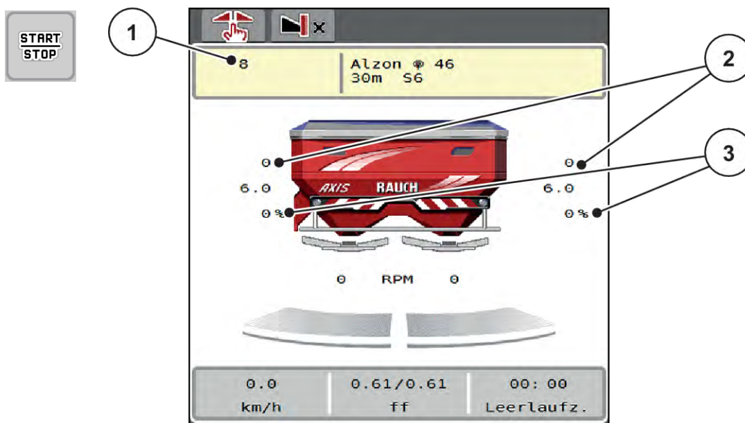
Kuva 50: Käyttökuva, MAN-asteikko
