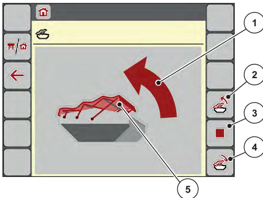
Kuva 30: Suojapeitteen valikko
