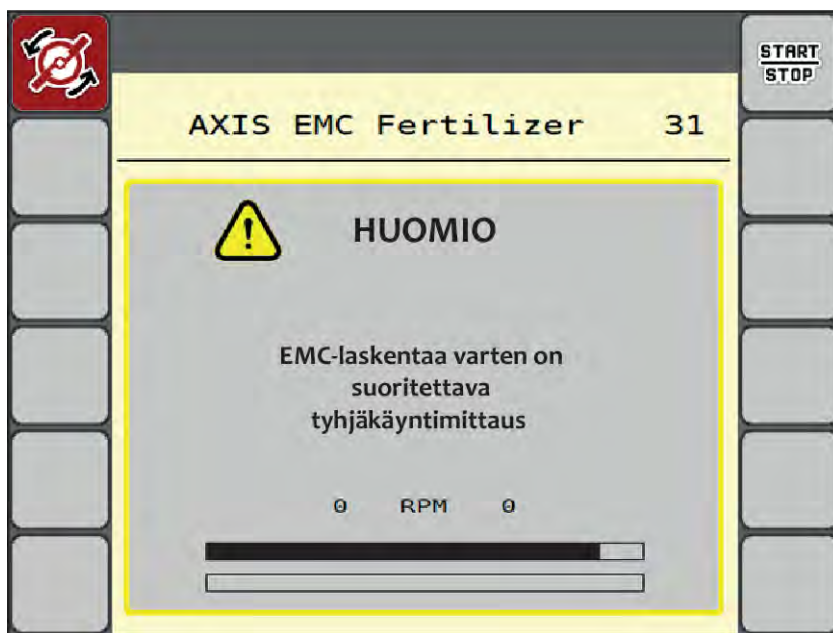
Kuva 44: Tyhjäkäyntimittauksen hälytysnäyttö
