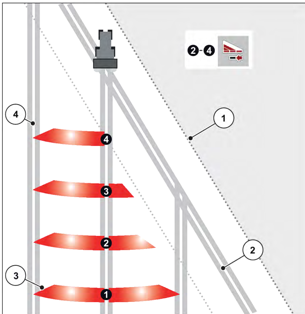
Kuva 40: Automaattinen osaleveyskytkin
