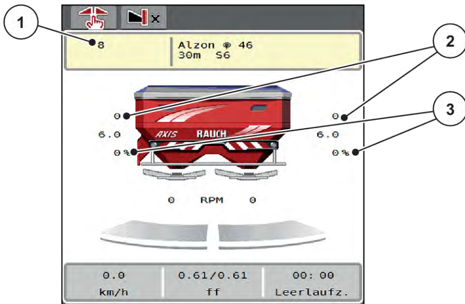
Kuva 46: Käyttökuva, MAN-asteikko
