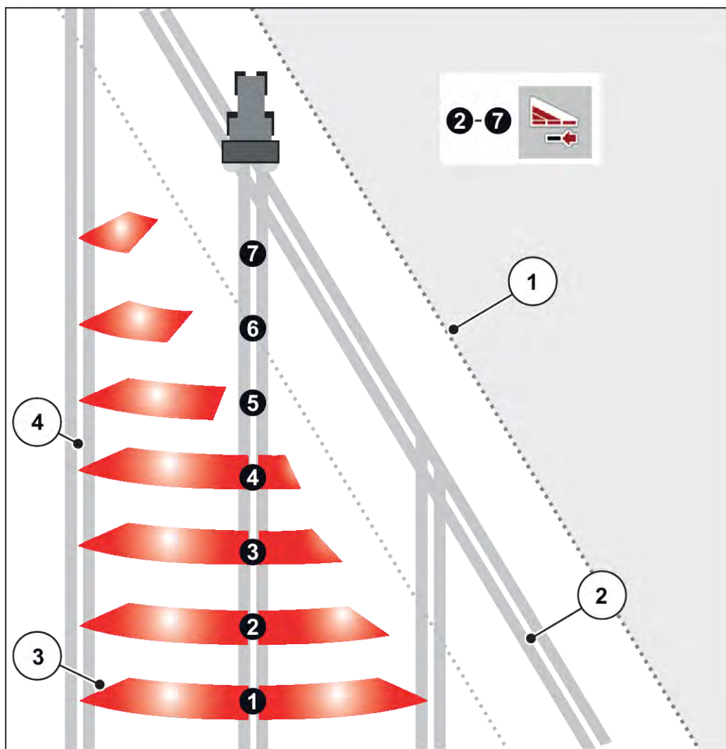
Kuva 42: Automaattinen osaleveyskytkin
