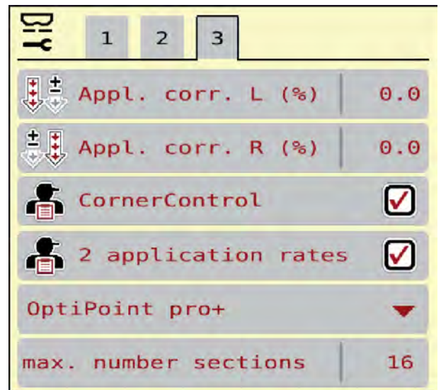
III. 26: Menu Impostaz. macchina, scheda 3
