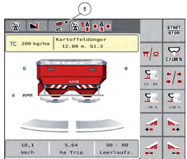
III. 32: Simbolo HillControl nella schermata di lavoro
