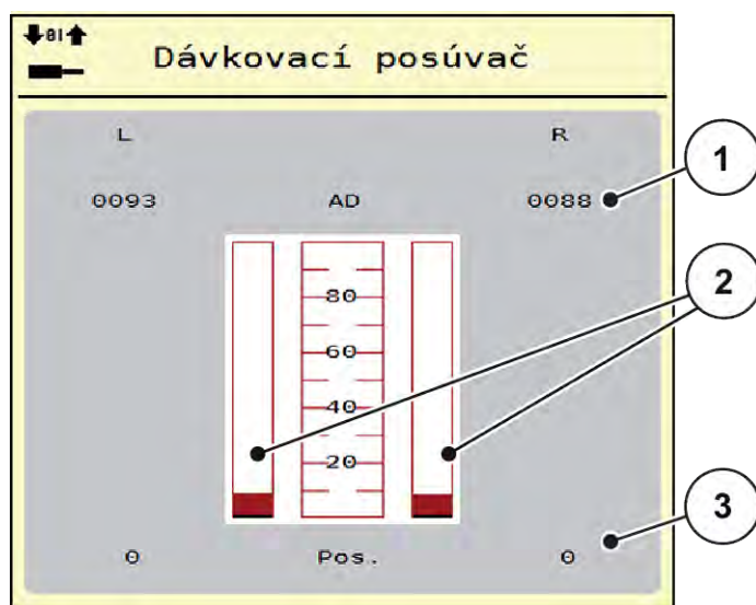
Obr. 24: Test/diagnostika; príklad: Dávkovací posúvač
