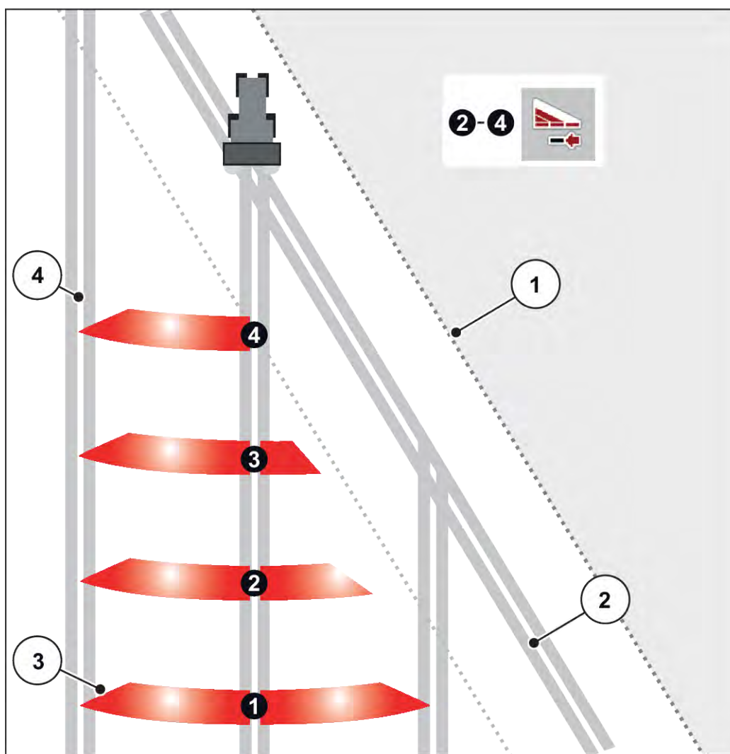
Obr. 40: Automatické spínanie čiastočnej šírky
