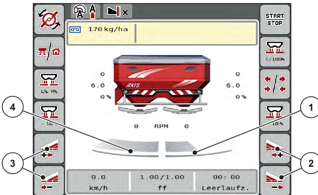
Obr. 39: Prevádzková obrazovka: Čiastočné šírky so 4 stupňami
