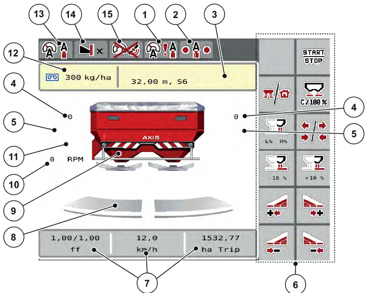
Obr. 1: Displej riadenia stroja AXIS-H
