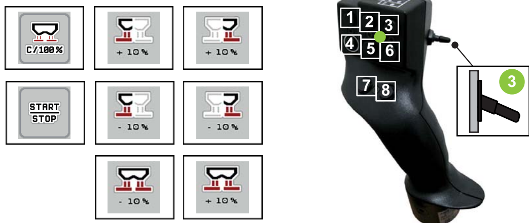
Bilde 4.24: Tastetilordning, nivå 3 (LED er grønn)
