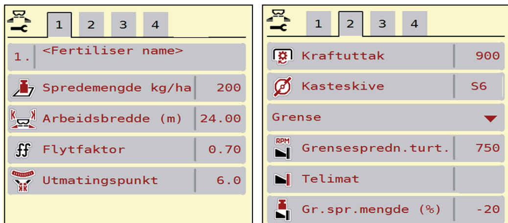
Bilde 4.3: Menyene Gjødseleinstillinger AXIS-M , fane 1 og 2
