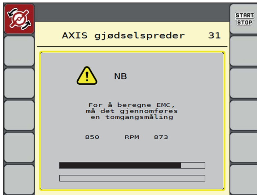
Bilde 5.6: Alarmvisning tomgangsmåling
