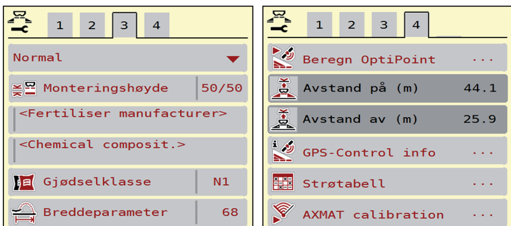
Bilde 4.4: Menyene Gjødseleinstillinger, fane 3 og 4
