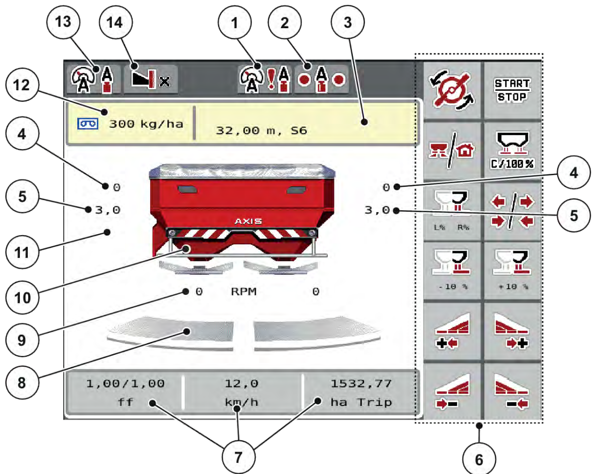
Ilust. 2: Pantalla del sistema de control de la máquina AXIS-M
