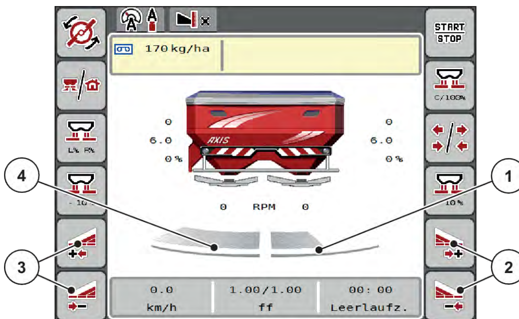
Ilust. 39: Pantalla de funcionamiento: Anchuras parciales con 4 niveles
