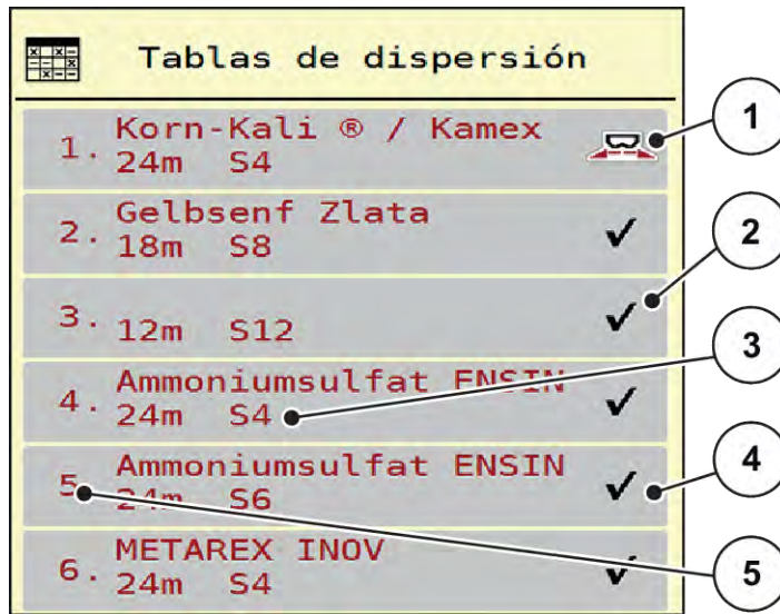
Ilust. 17: Menú Tablas de dispersión
