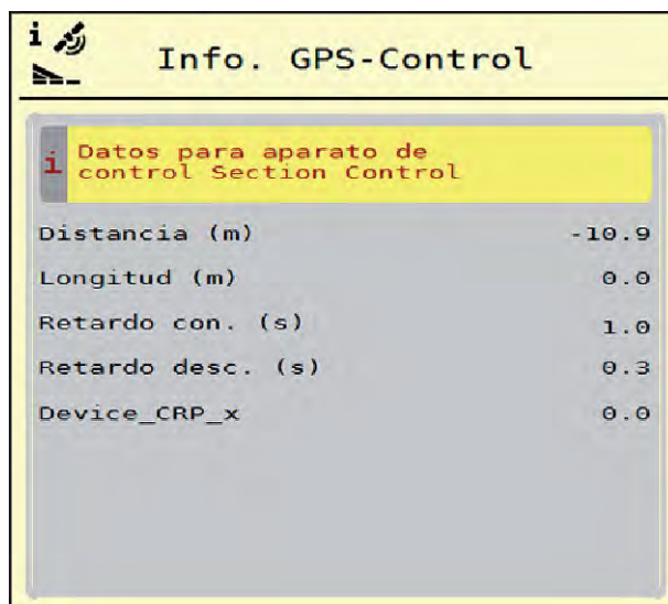
Ilust. 16: Menú Info. GPS-Control
