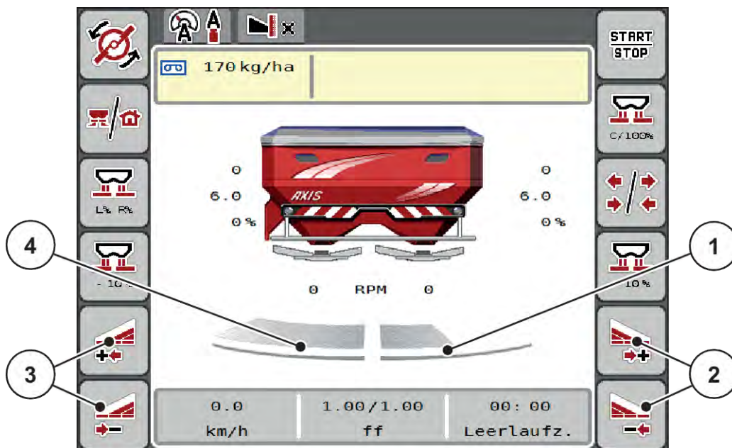
Ilust. 41: Pantalla de funcionamiento: Conmutación continua de anchuras parciales
