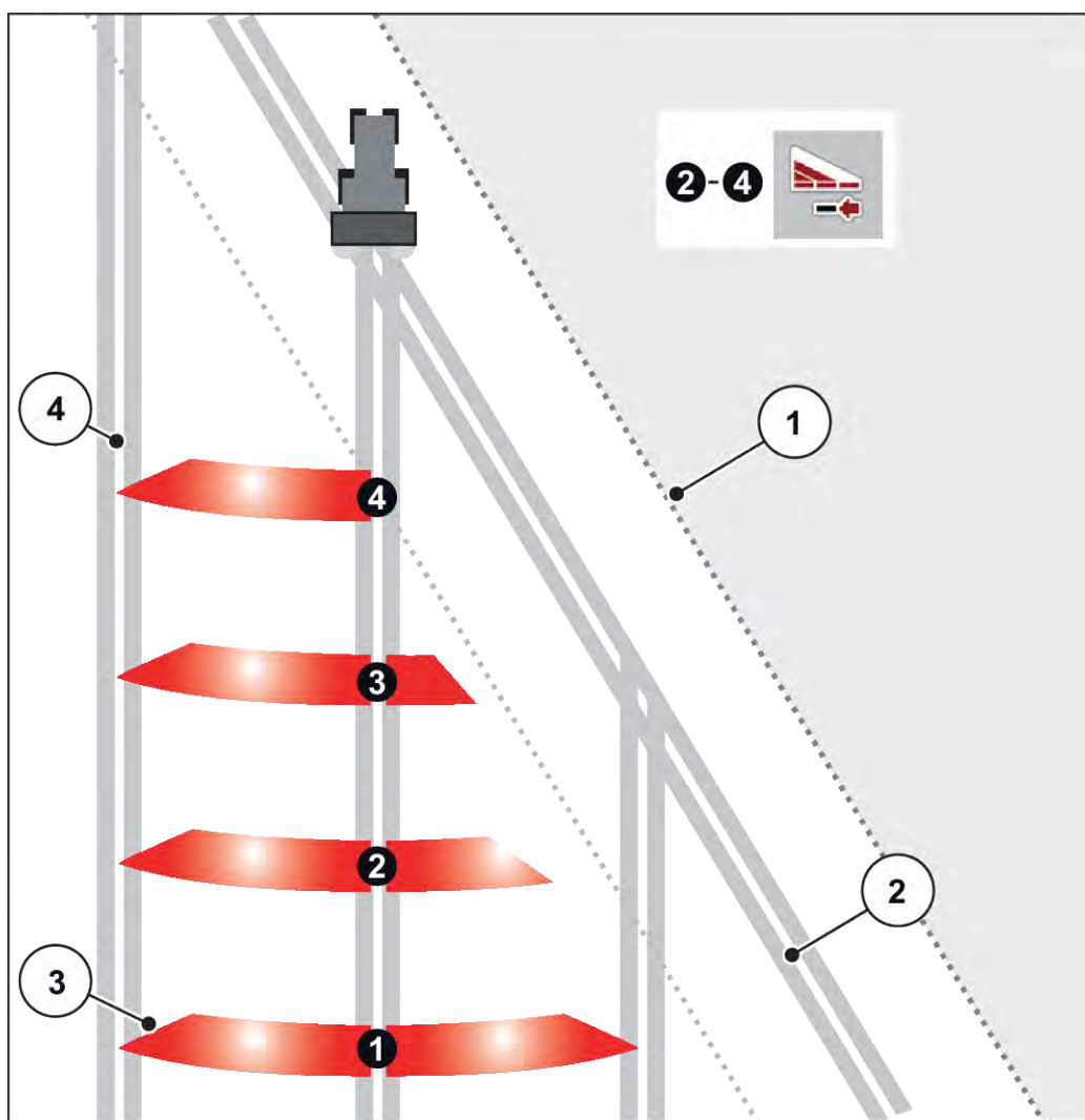
Ilust. 40: Conexión de anchuras parciales automática
