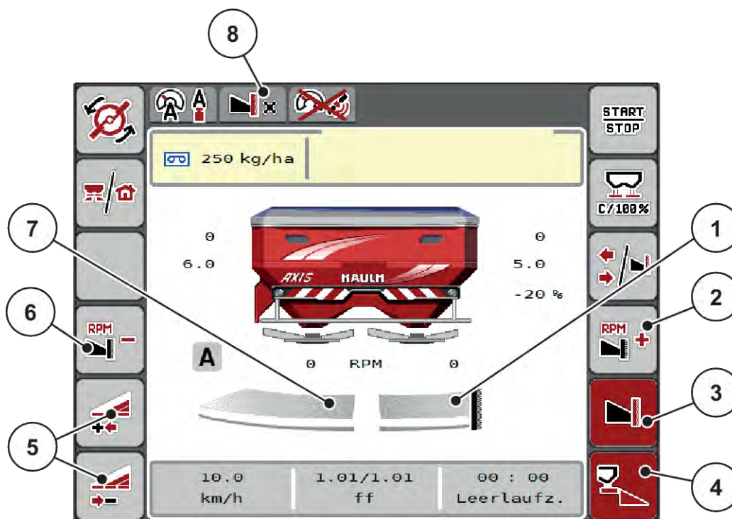
Ilust. 43: Pantalla de funcionamiento de una anchura parcial izquierda, lado de dispersión límite derecho
