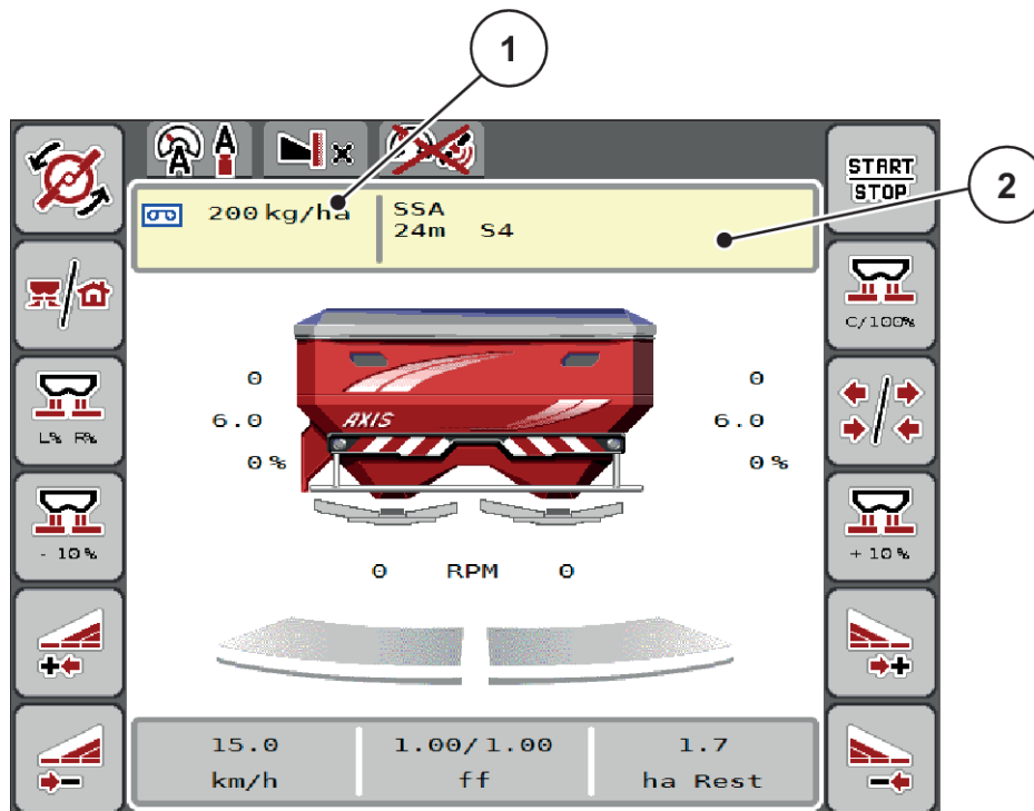
Ilust. 18: Administrar tabla de dispersión mediante pantalla táctil
