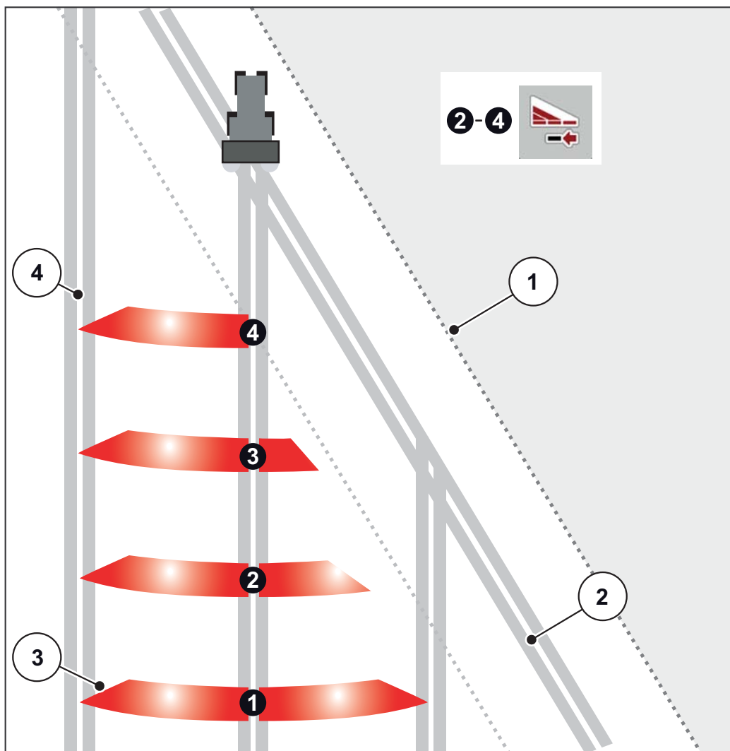
Imagen 5.4: Conexión de anchuras parciales automática (AXIS-M 20.2)
