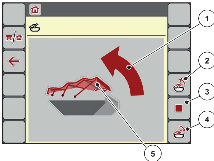
Imagen 4.20: Menú Lona de cubierta
