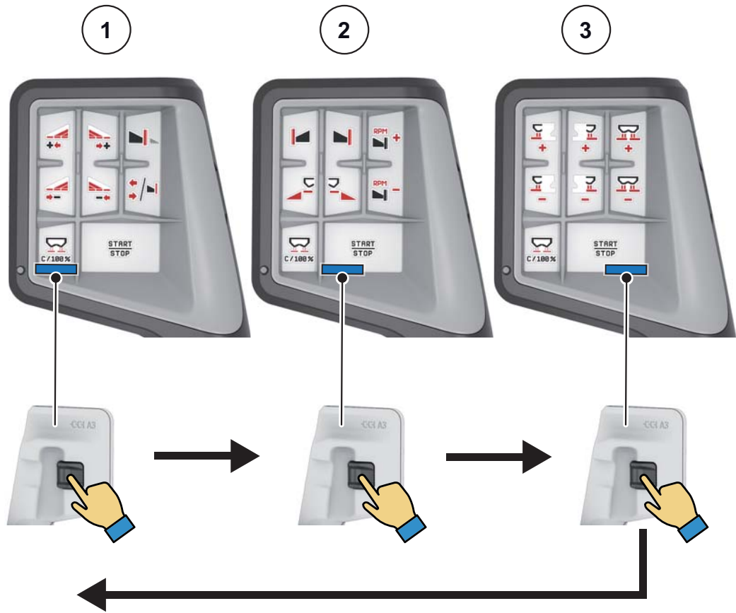
Imagen 4.22: Joystick CCI A3, visualización de niveles de mando
