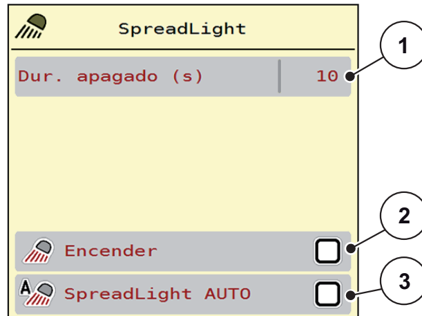
Imagen 4.19: Menú SpreadLight
