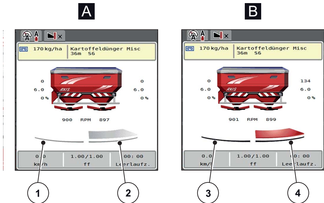
Bild 2.4: Visning av doseringsslidlägen
