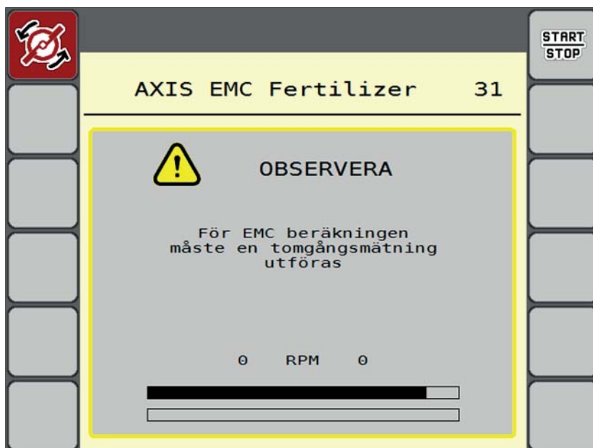
Bild 5.6: Alarmvisning under tomgångsmätning
