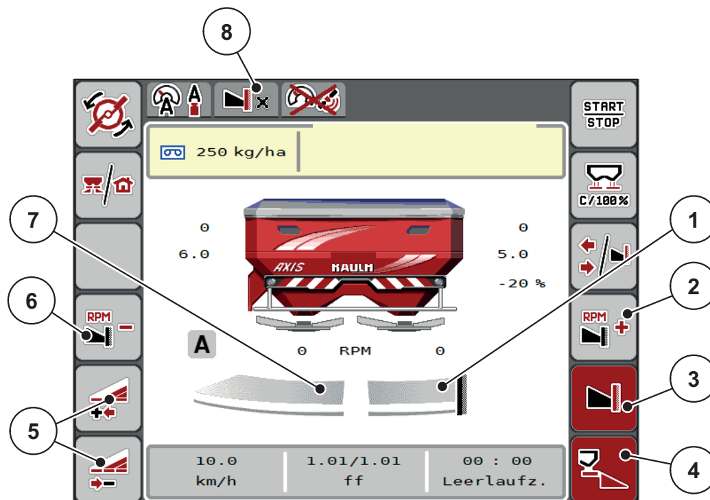
Bild 5.5: Driftsbild för en delbredd vänster, gränsspridningssida höger
