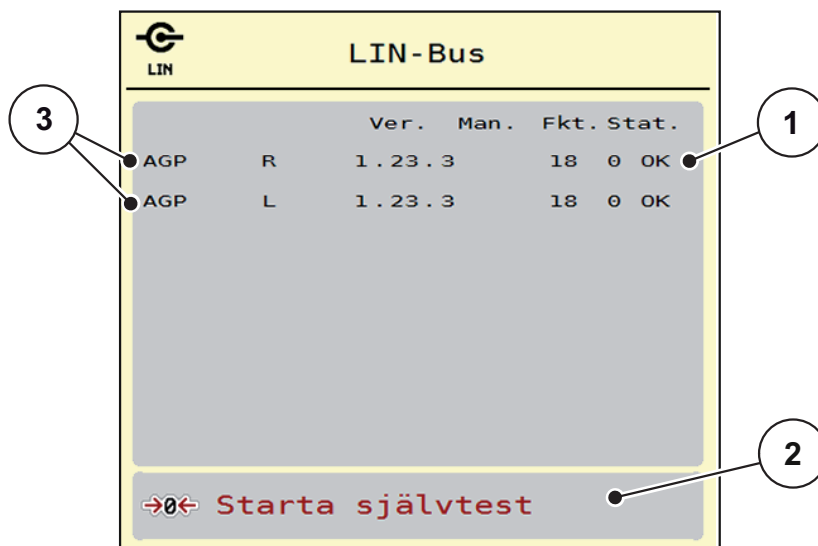
Bild 4.16: Test/diagnos; exempel: Linbus
