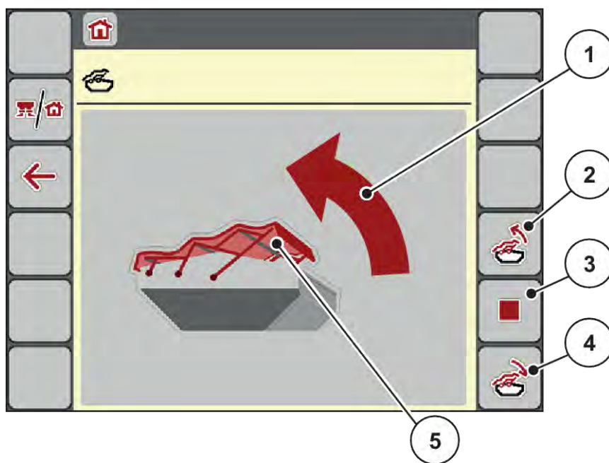
Фиг. 30: Меню Брезент
