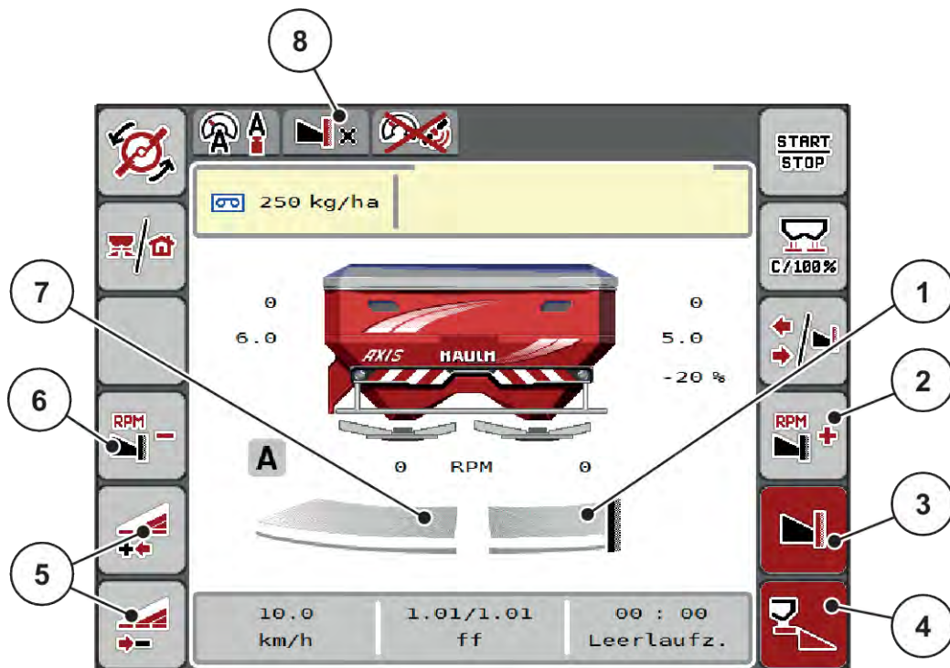
Фиг. 43: Работен екран една частична ширина отляво, страна с гранично разпръскване отдясно
