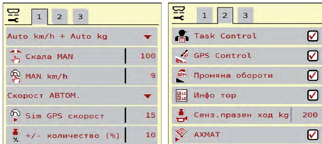
Фиг. 19: Меню Настройки машина, раздел 1 и 2
