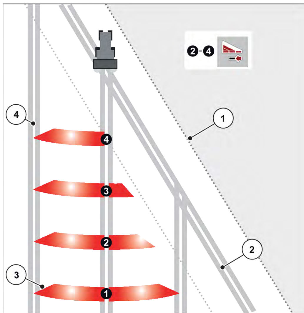
Фиг. 40: Автоматично превключване на частични ширини
