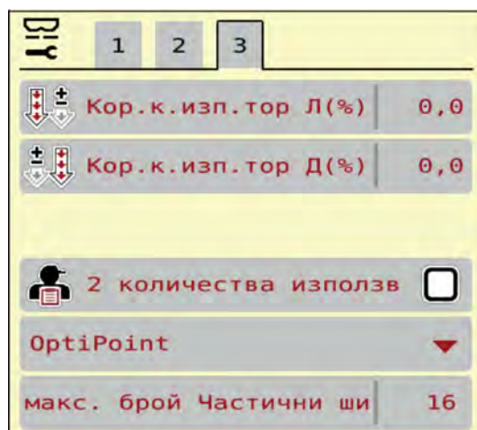
Фиг. 20: Меню Настройки машина, раздел 3
