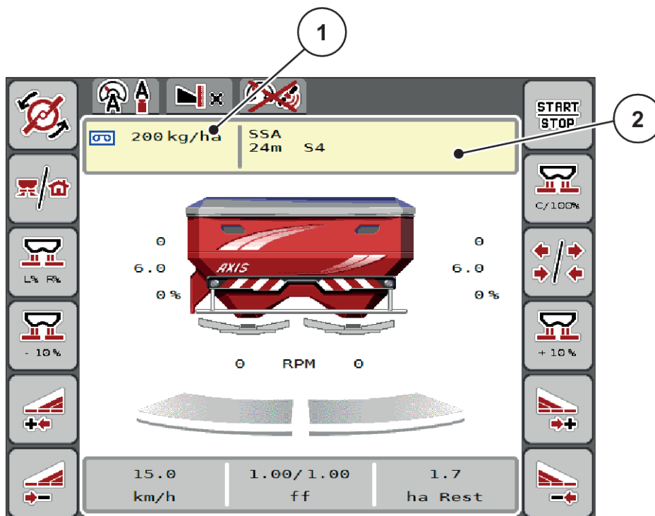
Фиг. 18: Управление на таблица на разпръскването от сензорния екран
