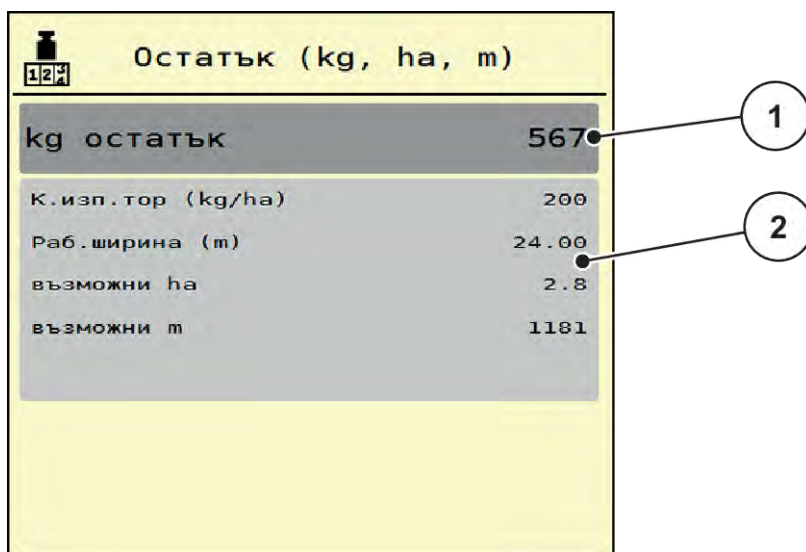
Фиг. 28: Меню Остатък (kg, ha, m)
