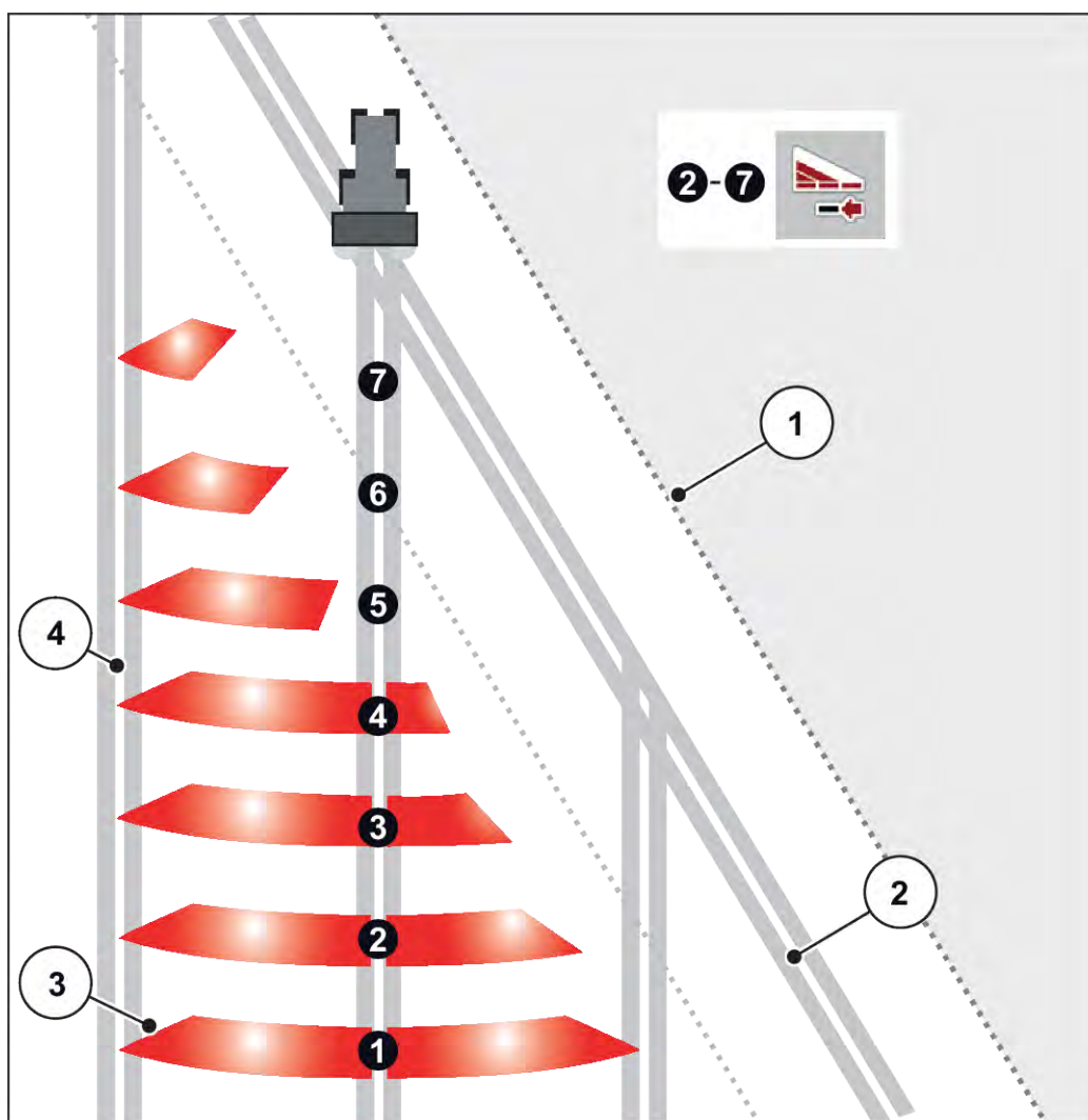
Фиг. 42: Автоматично превключване на частични ширини
