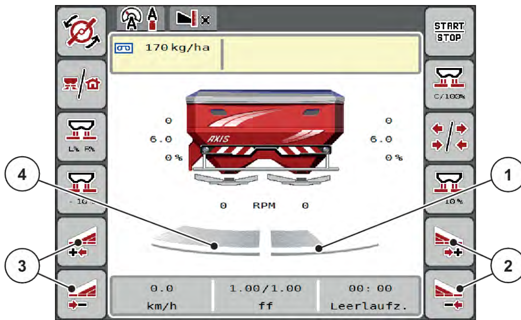
Фиг. 41: Работен екран: Плавно превключване на частични ширини
