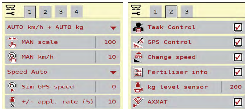
Att. 25: Izvēlnē Mašīnas iestatījums, 1. un 2. cilne
