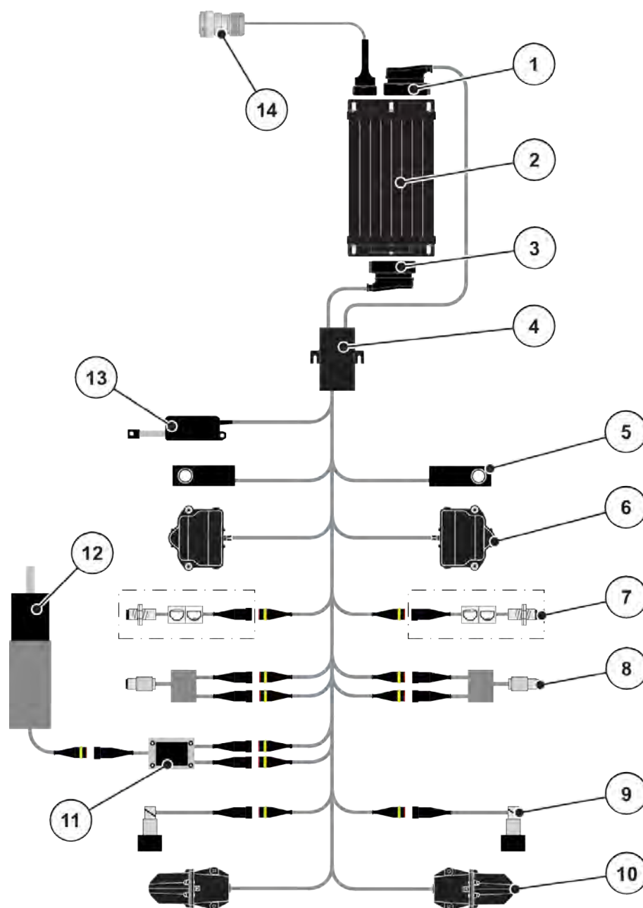
Att. 6: AXIS-H EMC: Shematiskis pieslēguma pārskats
