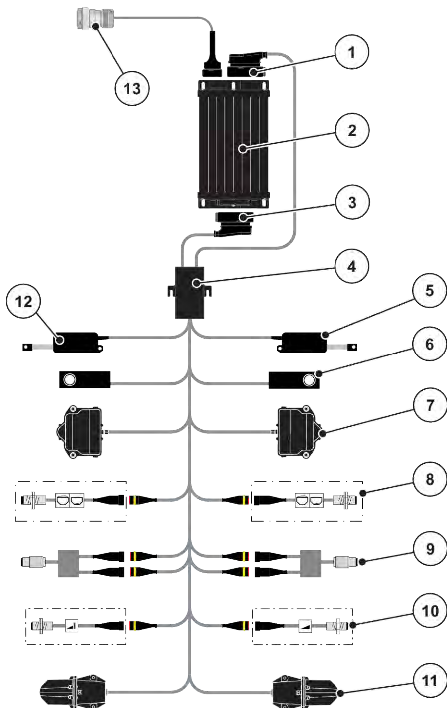
Att. 8: AXIS-M 30.2 EMC, AXIS-M 50.2: Shematiskis pieslēguma pārskats
