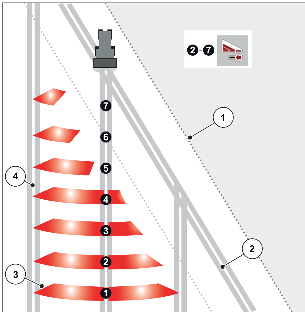
Rysunek 5.4: Automatyczne przełączenie szerokości częściowej
