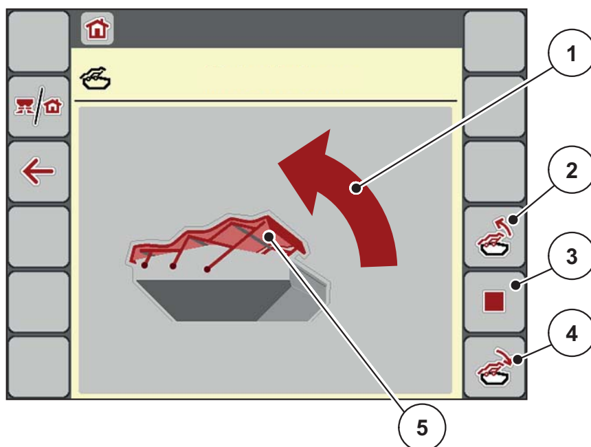
Rysunek 4.21: Menu Plandeka
