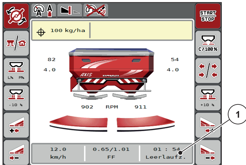
Rysunek 5.7: Wskazanie pomiaru biegu jałowego na ekranie roboczym [1] Czas do następnego pomiaru biegu jałowego
