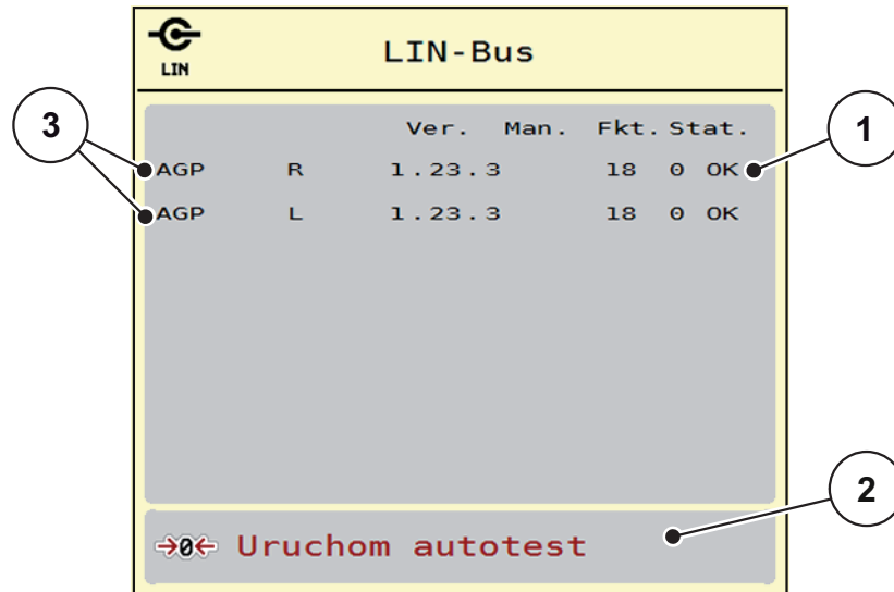
Rysunek 4.16: Test/diagnostyka; przykład: Linbus
