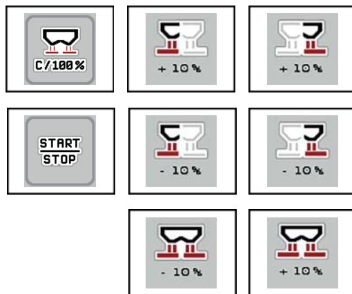
Rysunek 4.24: Przyporządkowanie przycisków, poziom 3 (dioda zielona)
