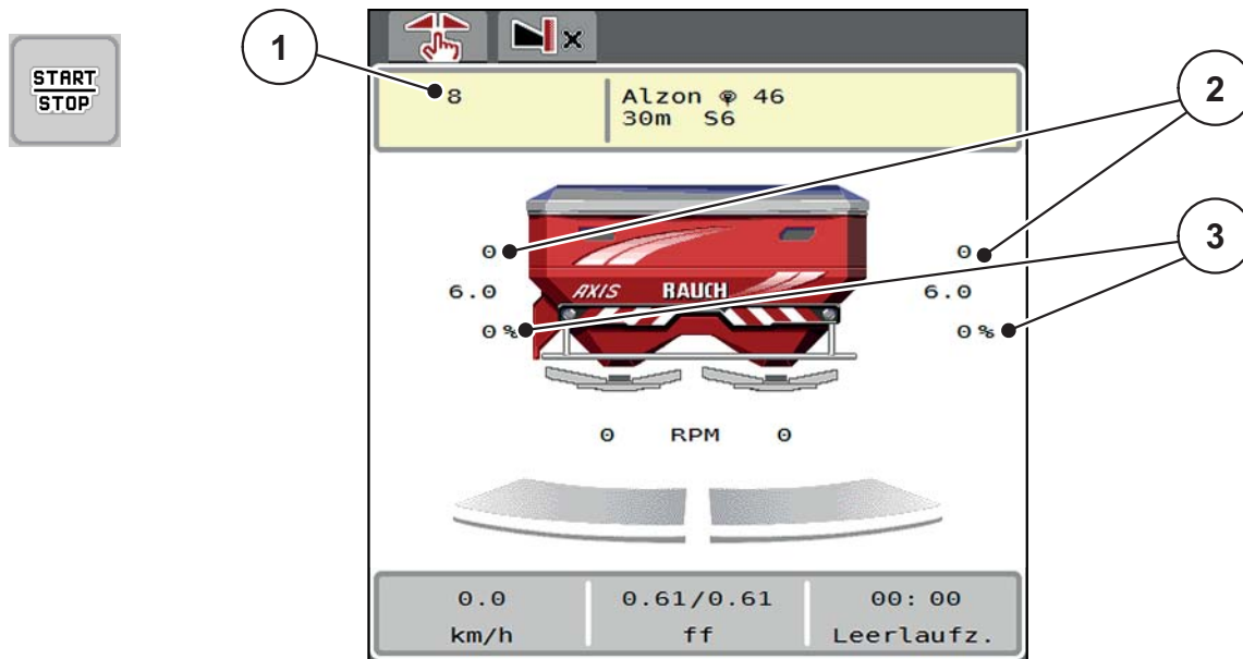
Rysunek 5.8: Ekran roboczy Skala MAN
