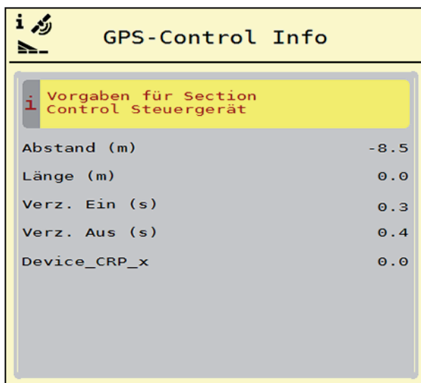
Rysunek 4.8: Menu GPS-Control Info
