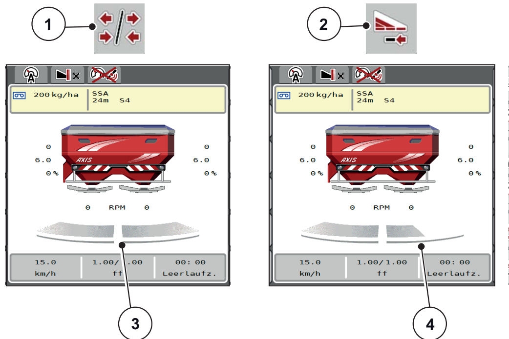
Rysunek 2.5: Wskazanie stanów szerokości częściowych
