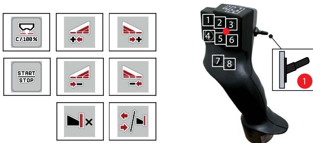
Rysunek 4.22: Przyporządkowanie przycisków, poziom 1 (dioda czerwona)
