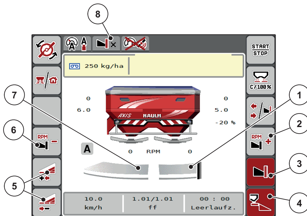
Rysunek 5.5: Ekran roboczy z jedną szerokością częściową po lewej stronie i wysiewem granicznym po prawej stronie
