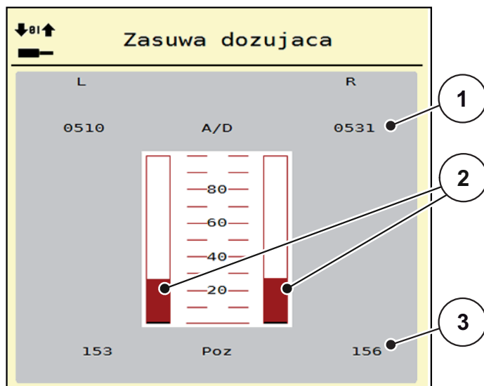
Rysunek 4.15: Test/diagnostyka; przykład: Zasuwa dozująca
