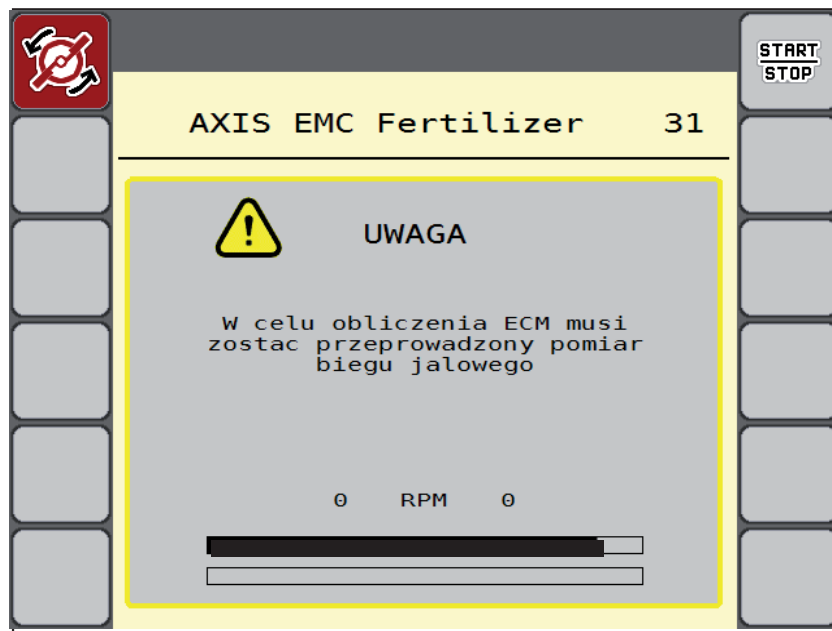
Rysunek 5.6: Wskazanie alarmów pomiaru biegu jałowego
