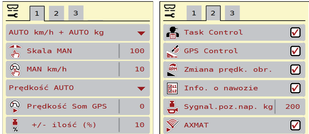
Rysunek 4.11: Menu Ustawienia maszyny, strona 1 i 2
