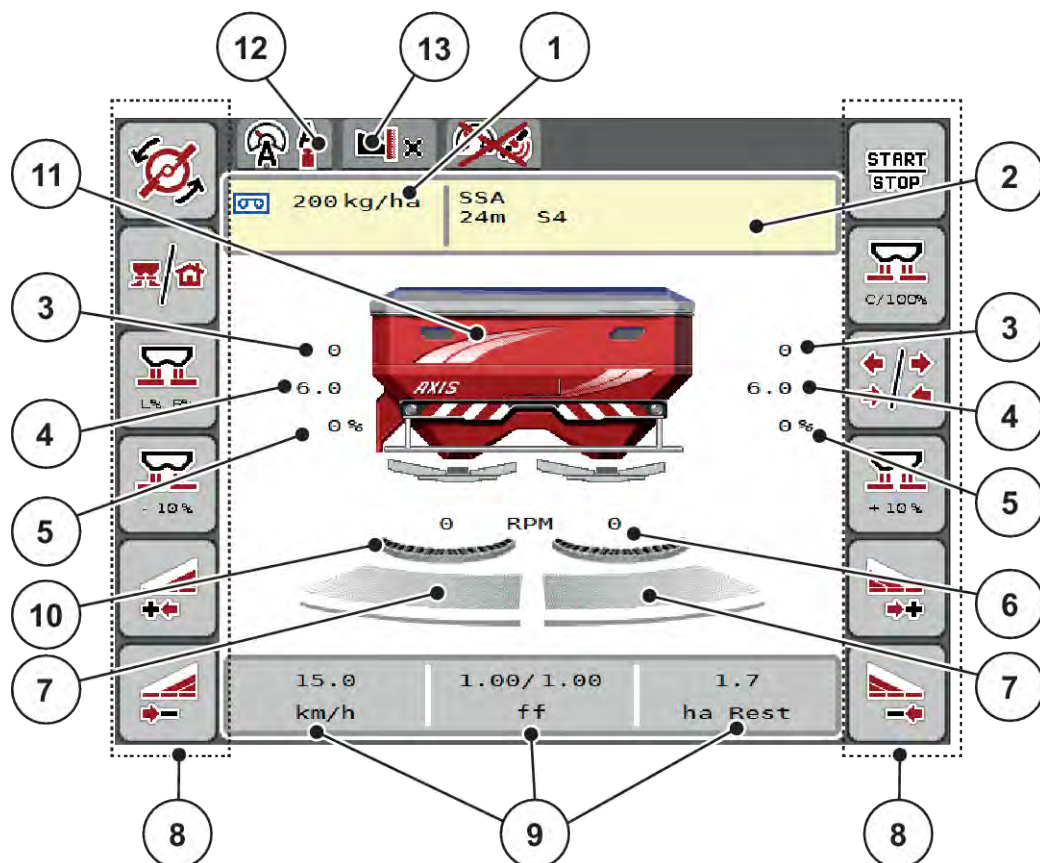
Fig. 1: Maskinstyringens display
