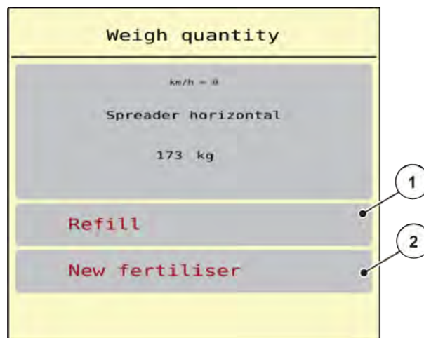
[1] Refill - Nouveau remplissage [2] New fertiliser - Nouvel engrais
