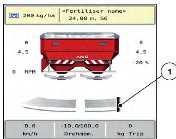
Fig. 42: Affichage TELIMAT
