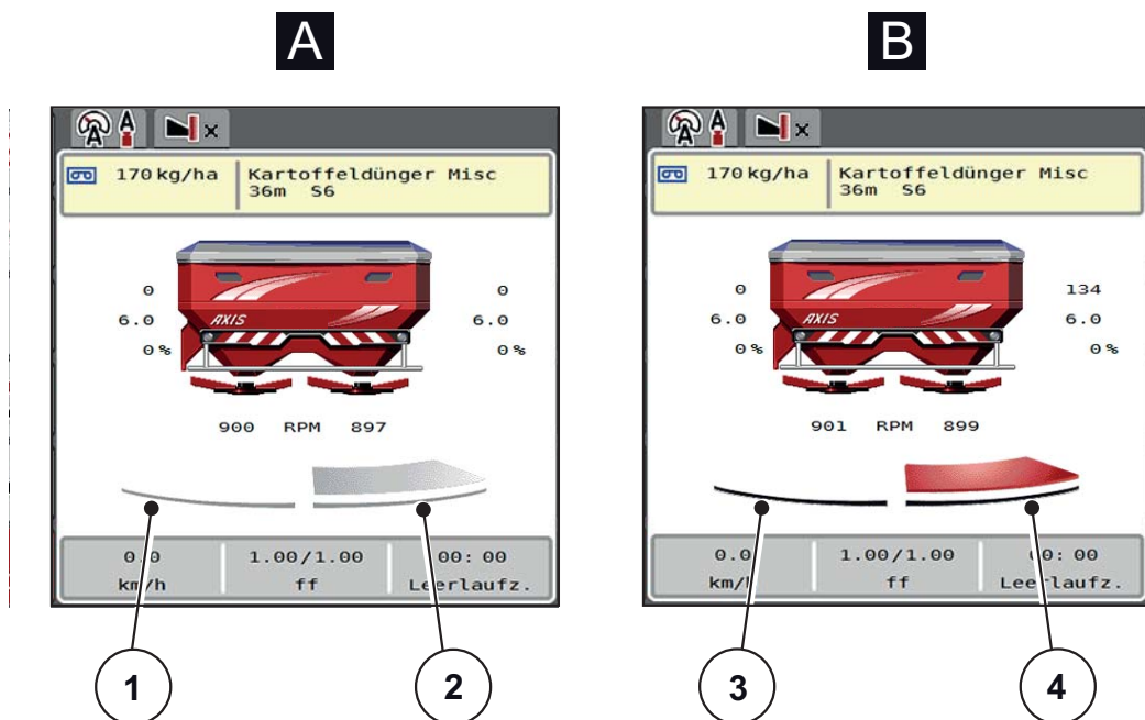
Figure 2.4 : Affichage des états de la vanne de dosage
