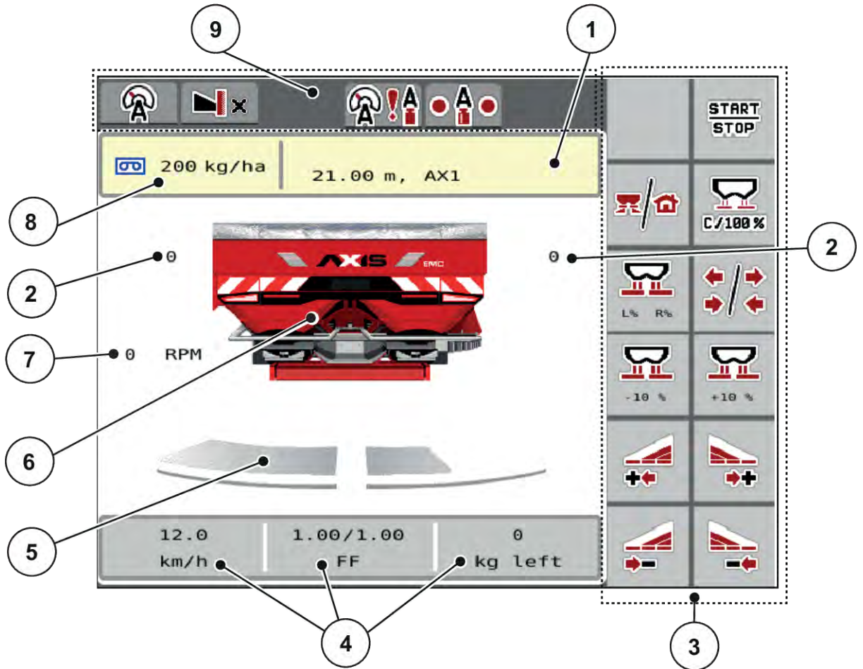
Şek. 2: AXIS 25 makine kumanda sisteminin ekranı
