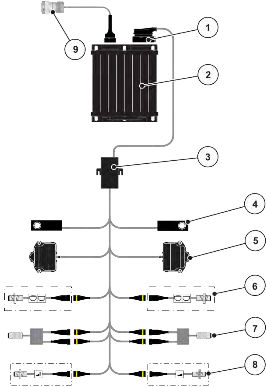
Şek. 6: AXIS 25: Şematik bağlantı özeti
