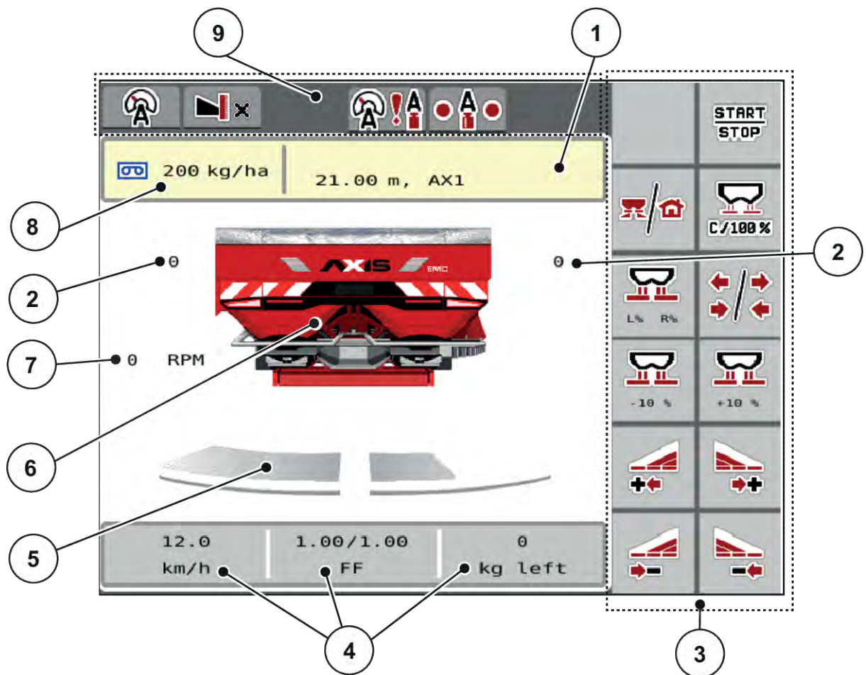
Pav. 2: Padargo valdymo sistemos AXIS 25 ekranas
