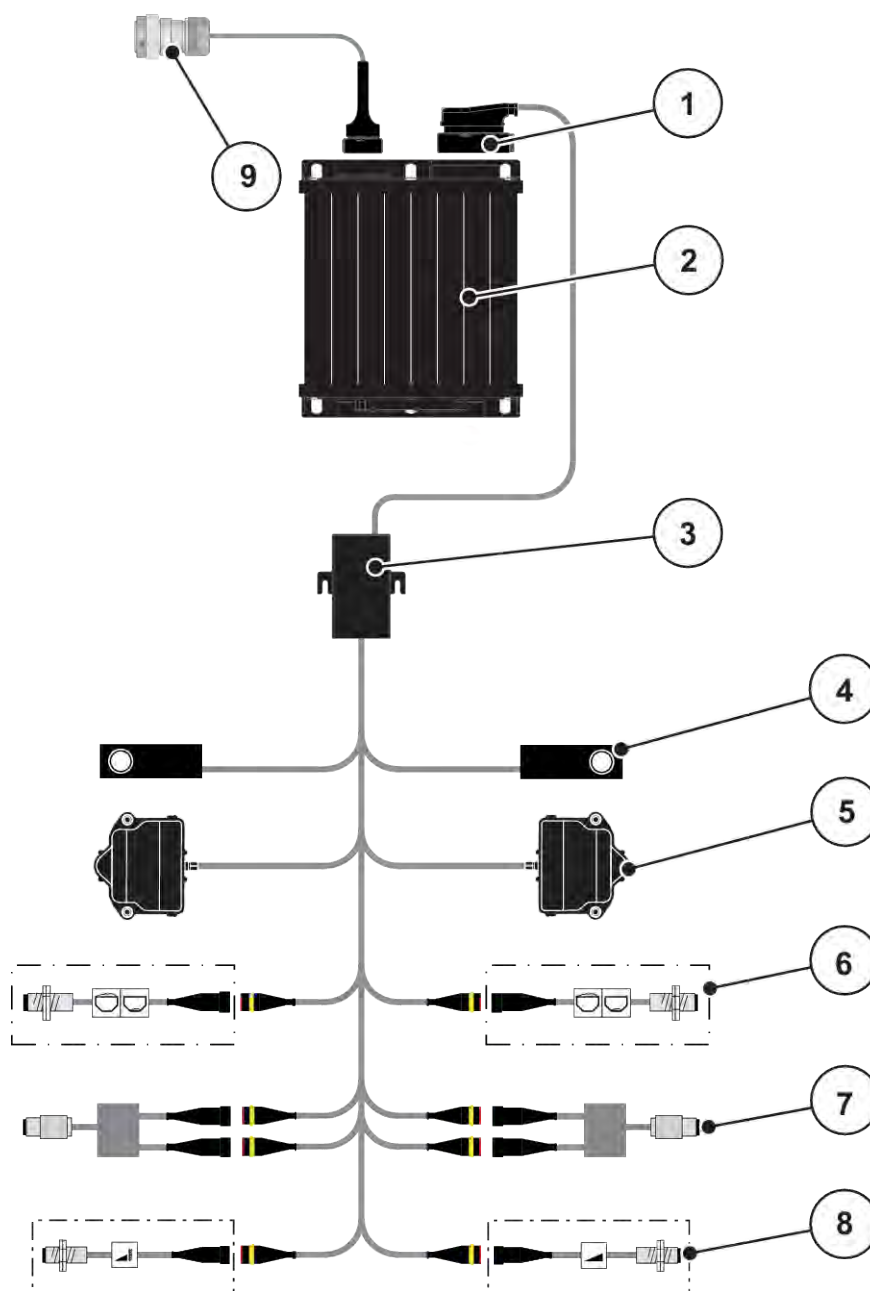
Pav. 6: AXIS 25: Prijungimo schemos apžvalga
