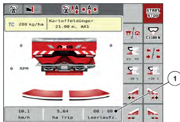
Att. 31: Tukšgaitas mērīšanas rādījums darba ekrānā
