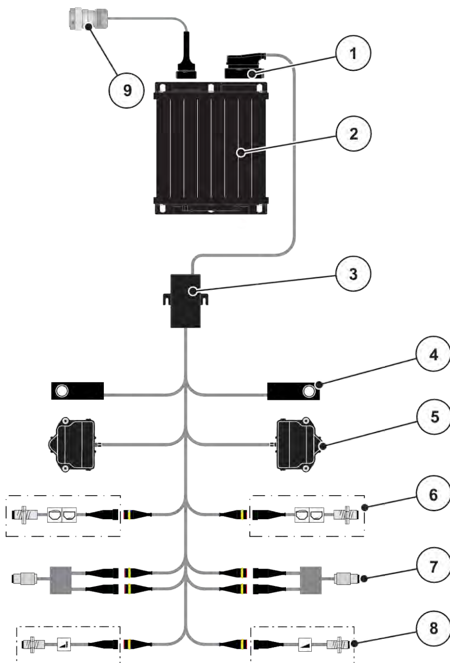
Att. 6: AXIS 25: Shematiskais pieslēgšanas pārskats
