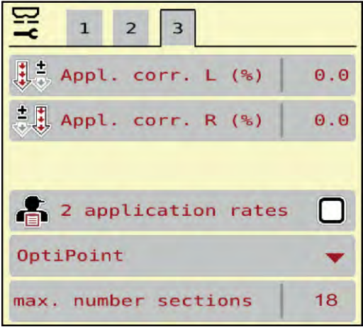
Afb. 16: Menu Machine-instelling, tabblad 3
