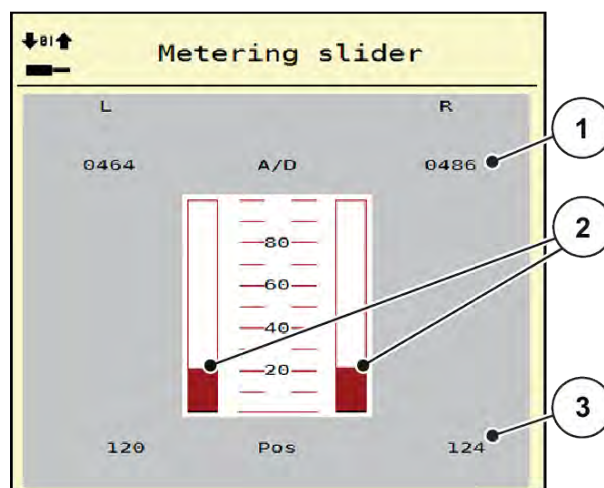
Afb. 20: Test/diagnose; voorbeeld: Metering slider - Doseerschuij
