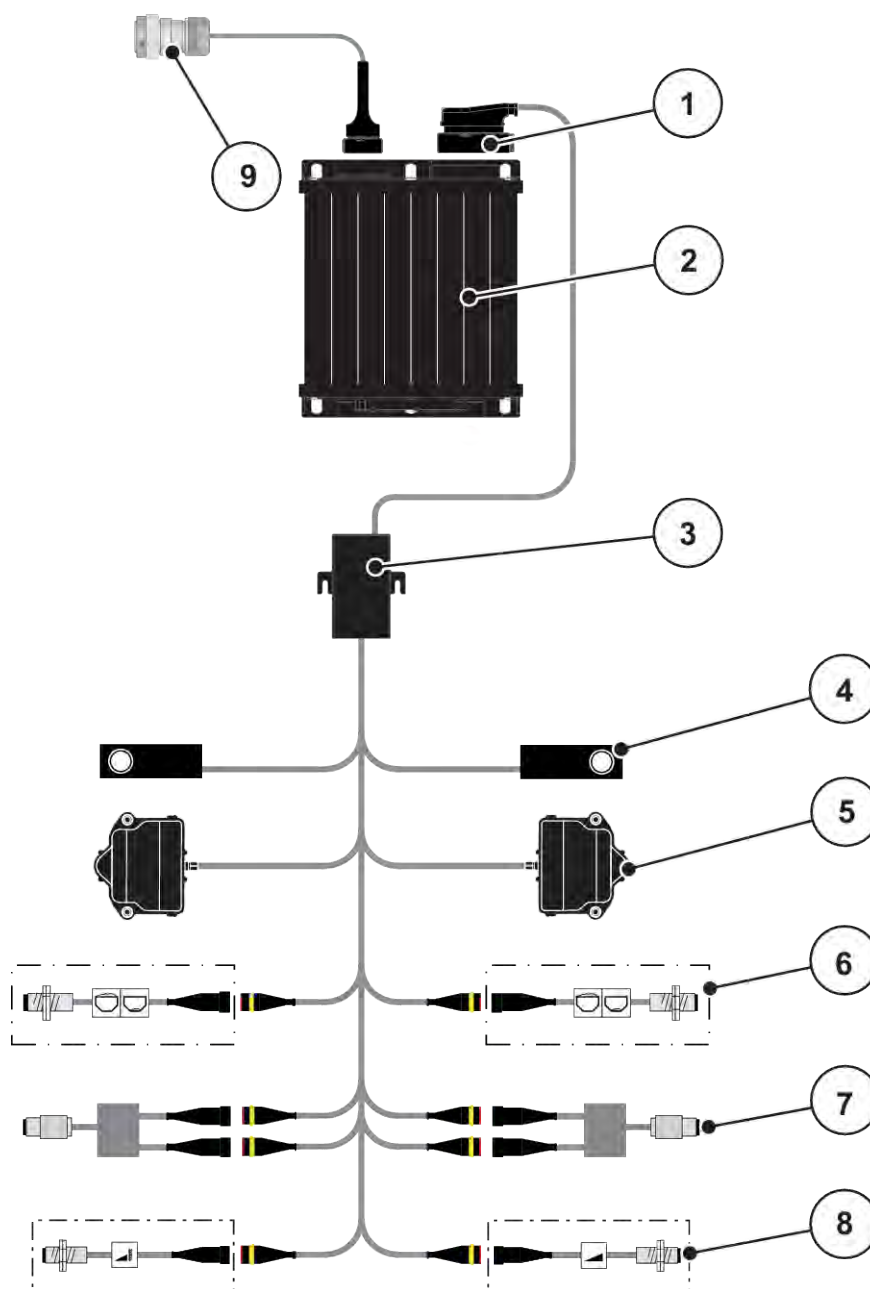
Afb. 6: AXIS 25: Aansluitschema
