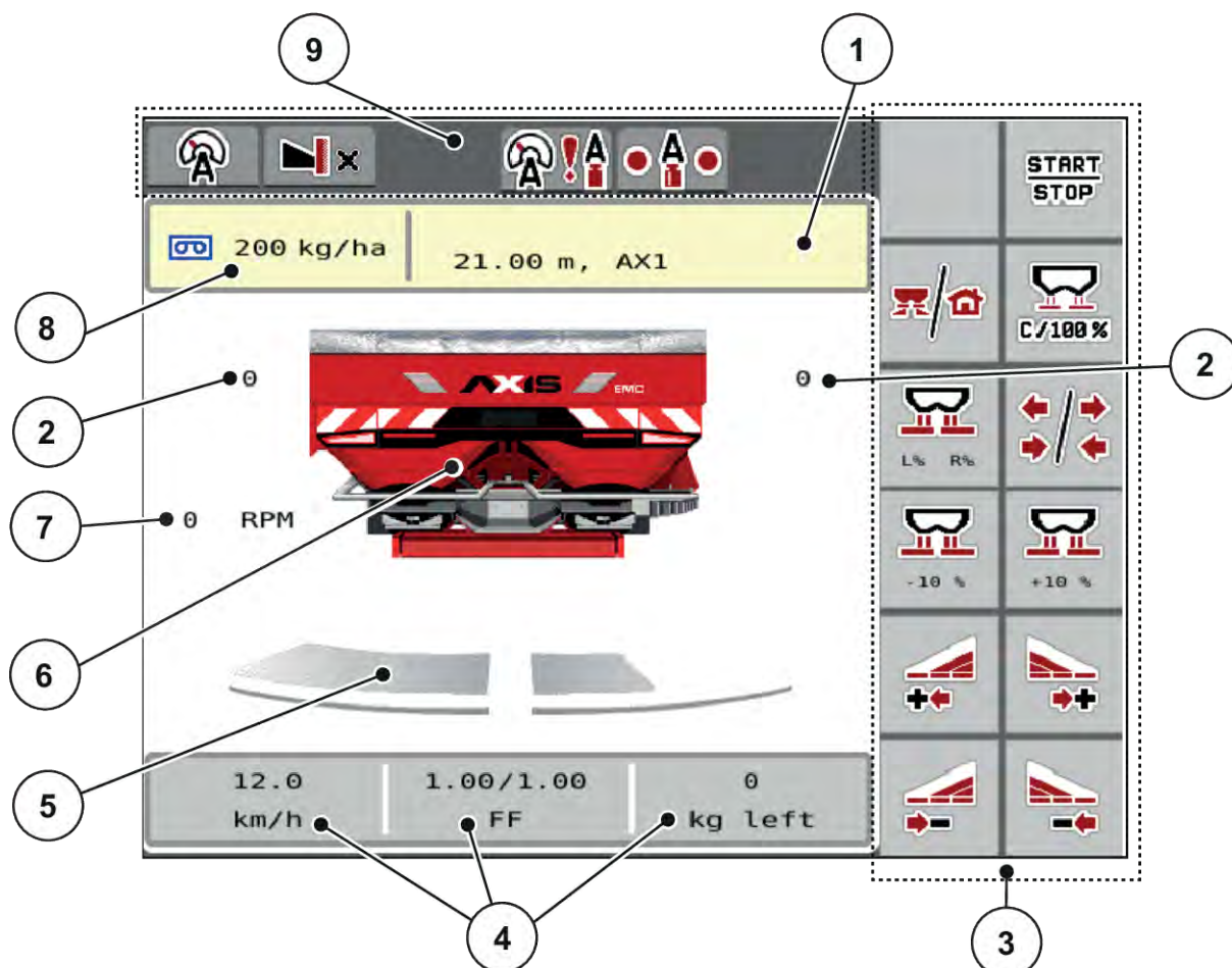
Sl. 2: Zaslón upravljačkog uređaja stroja AXIS 25
