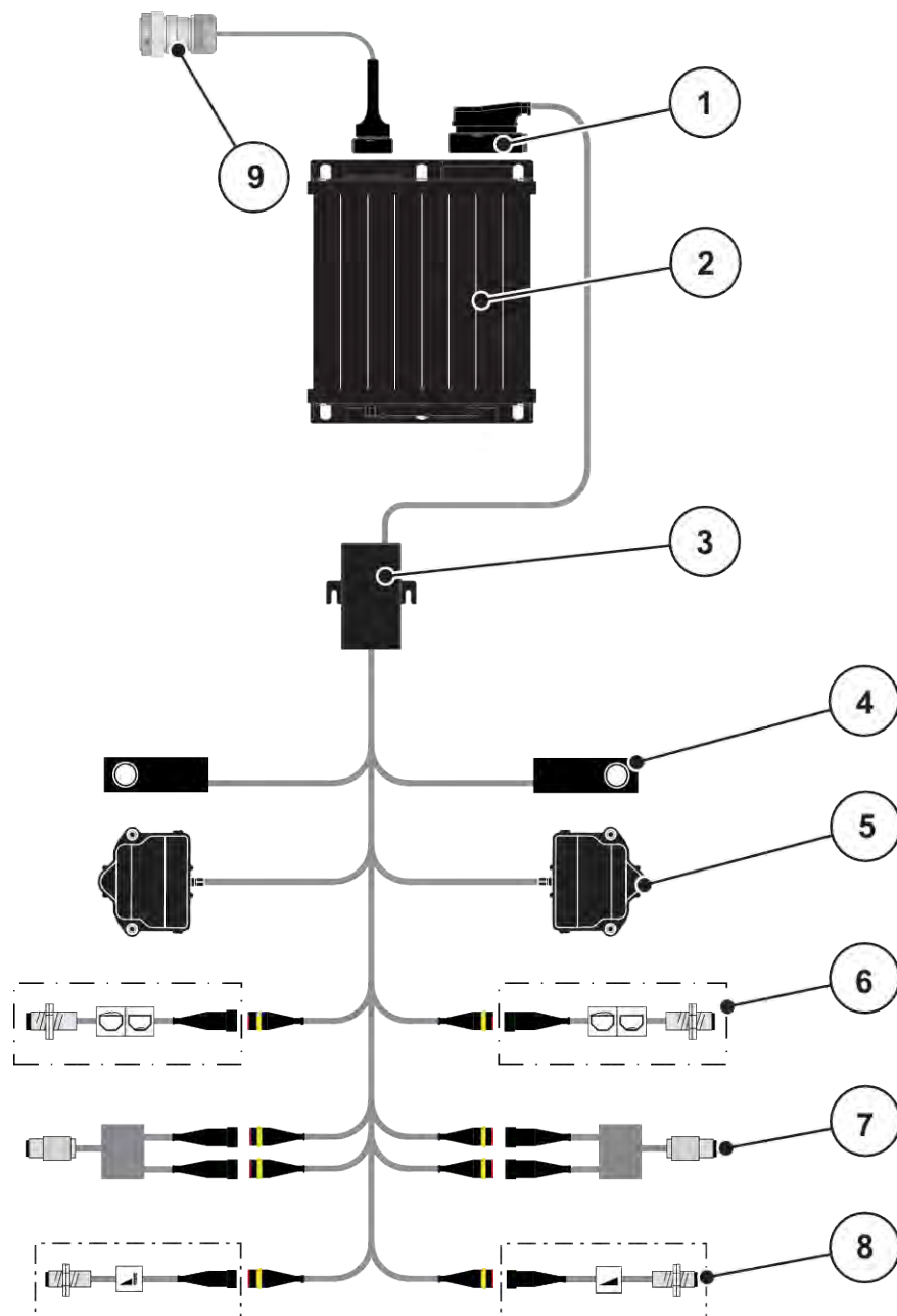
Abb. 6: AXIS 25: Schematische Anschlussübersicht
