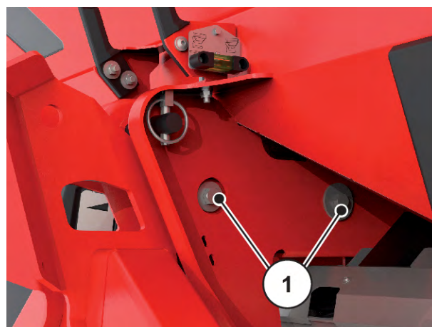
Sl. 44: Pričvršćivanje vučne šipke na okvir za vaganje
