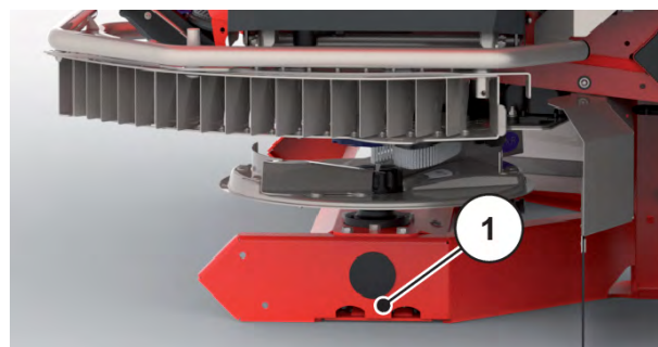
Sl. 49: Položaj otvora za čišćenje
