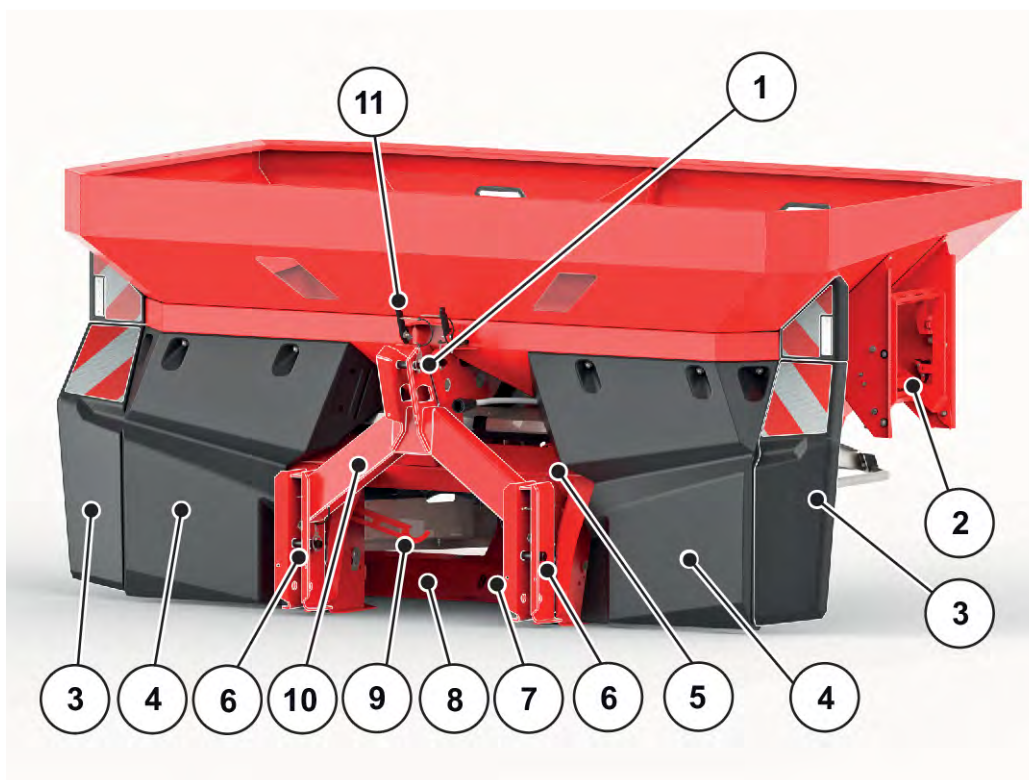
Sl. 6: Pregled sklopova: Prednja strana
