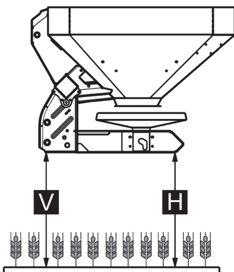
Sl. 22: Maksimalna dopuštena montažna visina za normalnu i kasnu gnojidbu
