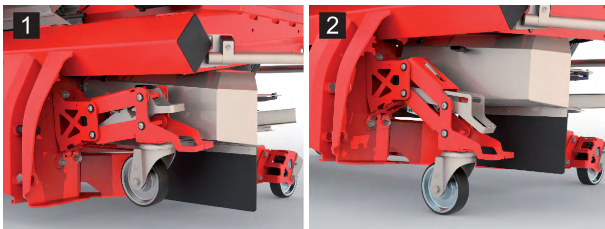
Sl. 12: Kotač za odlaganje sprijeda
