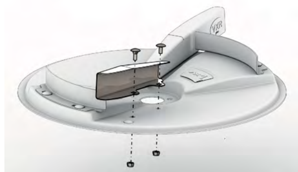
Sl. 55: Otpuštanje vijaka lopatice
