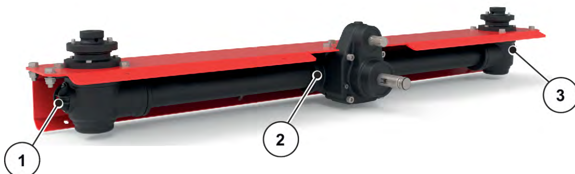
Sl. 8: Regulacija masenog protoka mjerenjem okretnog momenta diskova za rasipanje
