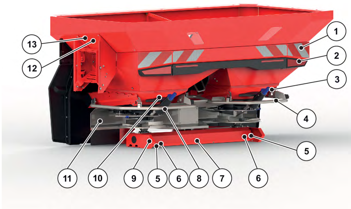
Sl. 3: Zaštitna oprema, naljepnica s upozorenjima i napomenama, stražnja strana
