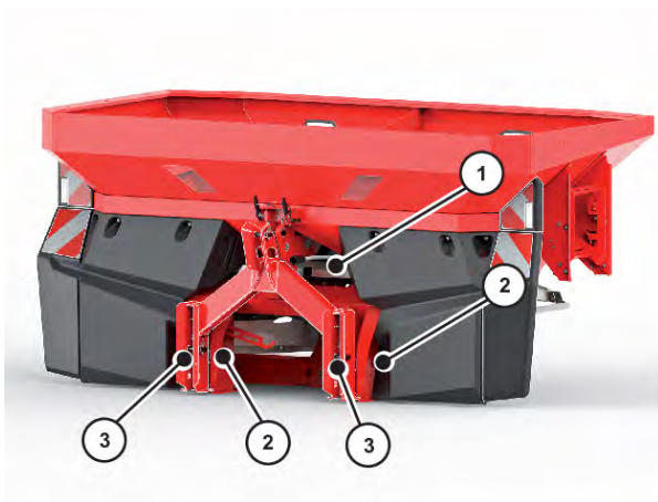
Sl. 48: Mjesta sprijeda i straga
