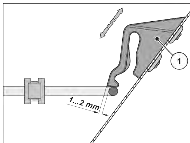
Sl. 47: Kontrolno mjerilo za provjeru funkcionalnosti blokade zaštitne rešetke
