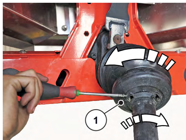
Sl. 15: Otpuštanje zaštite kardanskog vratila
