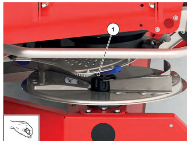
Sl. 33: Odvrtnje zaobljene slijepe matice
