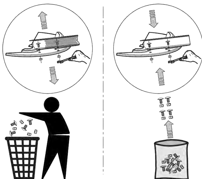
Sl. 56: Uporaba novih samoosiguravajućih matica
