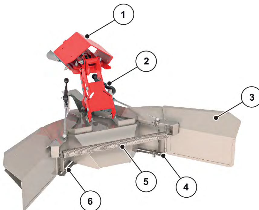
Рис. 22: Налаштування обмежувача ширини розкидання
