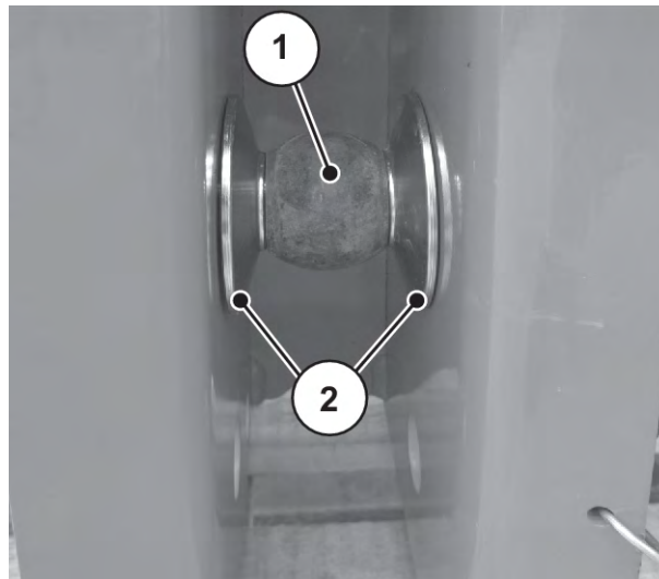
Рис. 16: Положення розпірних шайб під час установлення машини
