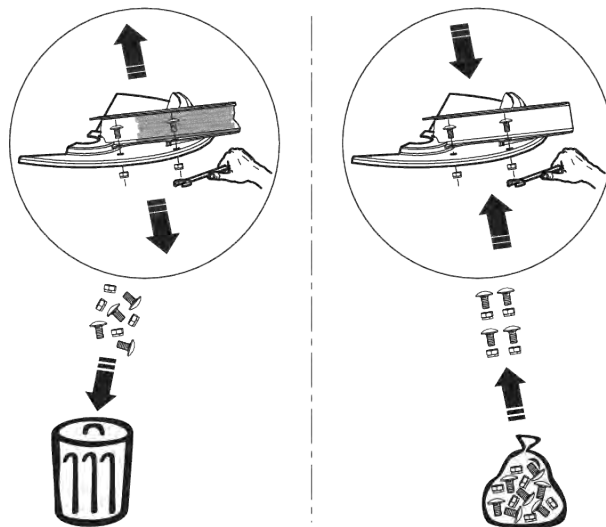
Рис. 58: Використовуйте нову самофіксуючу гайку
