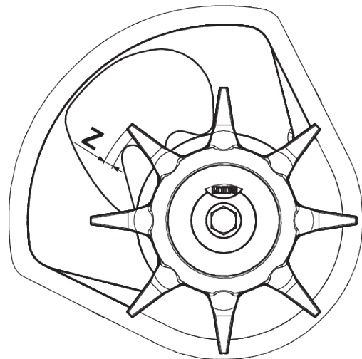
図 55: アジテーターターレットの磨耗範囲
