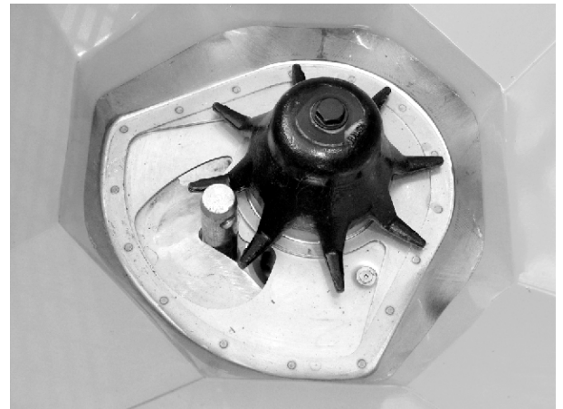
図 59: 調量アウトレットのロアリンクピン
