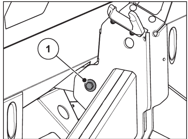
Kuva 47: Vetosauvan kiinnitys punnituskehukseen
