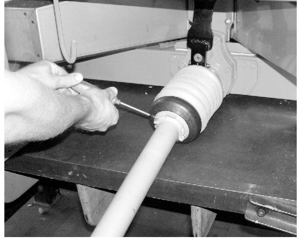
Şek. 14: Tahrik mili korumasını sabitleyin
