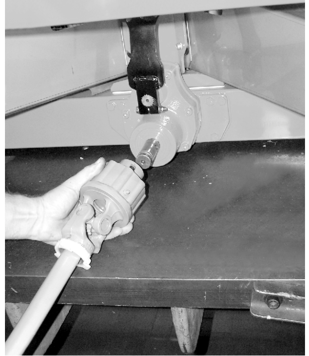
Şek. 11: Tahrik milini şanzıman miline monte edin
