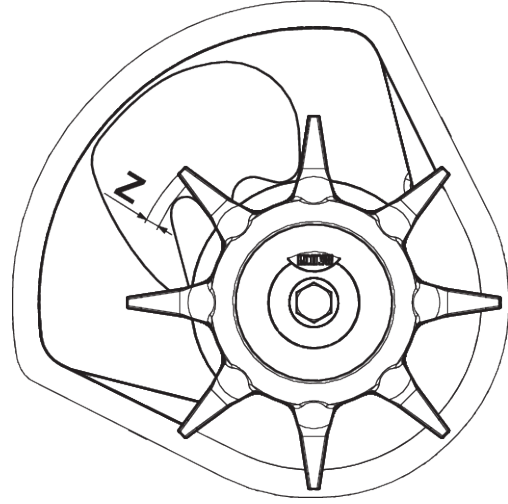
Şek. 55: Karıştırıcı kafasının aşınma bölgesi
