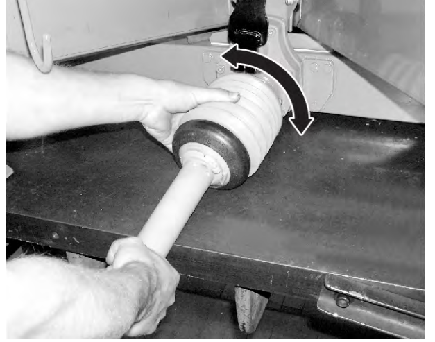
Şek. 13: Tahrik mili korumasını yerleştirin
