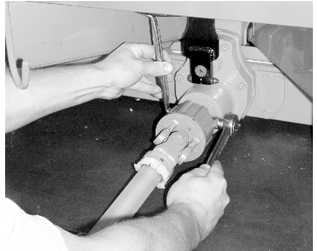
Şek. 12: Tahrik milini sabitleyin
