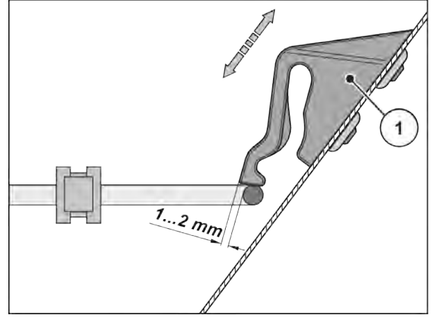
Şek. 51: Koruyucu ızgaranın fonksiyon kontrolü için kontrol göstergesi
