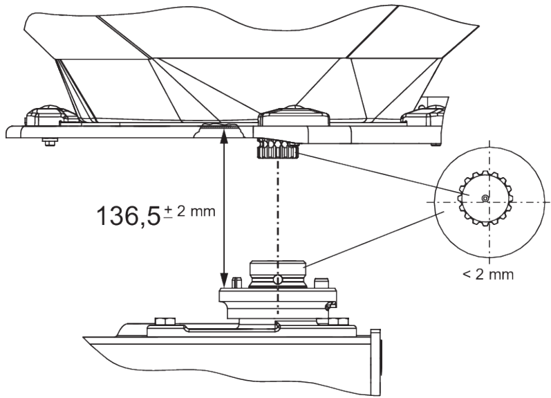
Şek. 53: Fırlatma diski göbeğinin konumunun kontrolü
