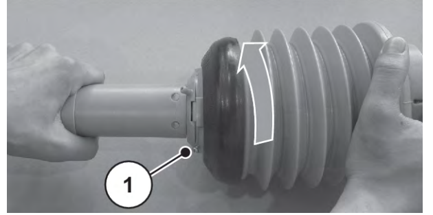
Şek. 10: Tahrik mili korumasını gevşetin
