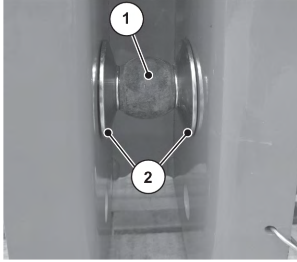
Şek. 16: Makine bağlantısında ara disklerin konumu
