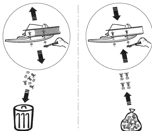
Sl. 58: Nato uporabite nove samovarovalne matice.
