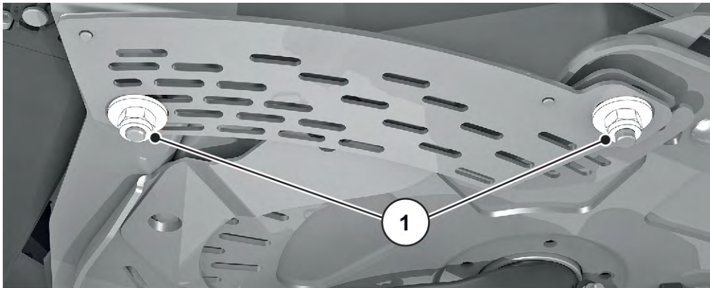
Sl. 61: Pritrdilni vijaki skale
