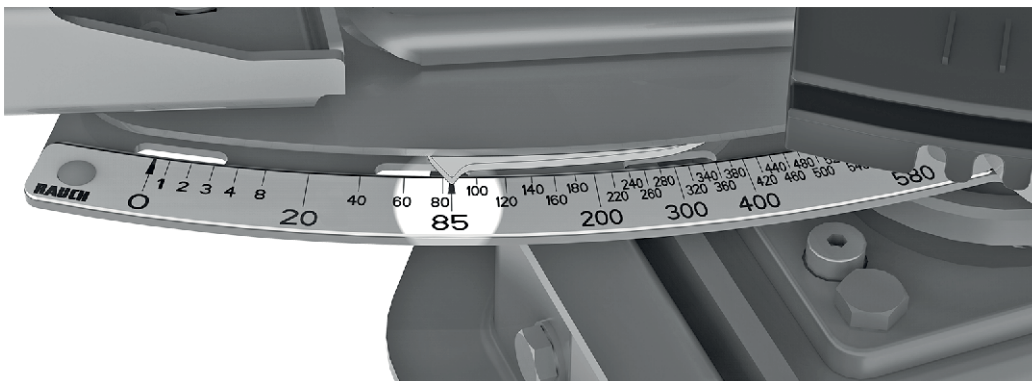
Sl. 62: Kazalec dozirnega drsnika na vrednosti 85
