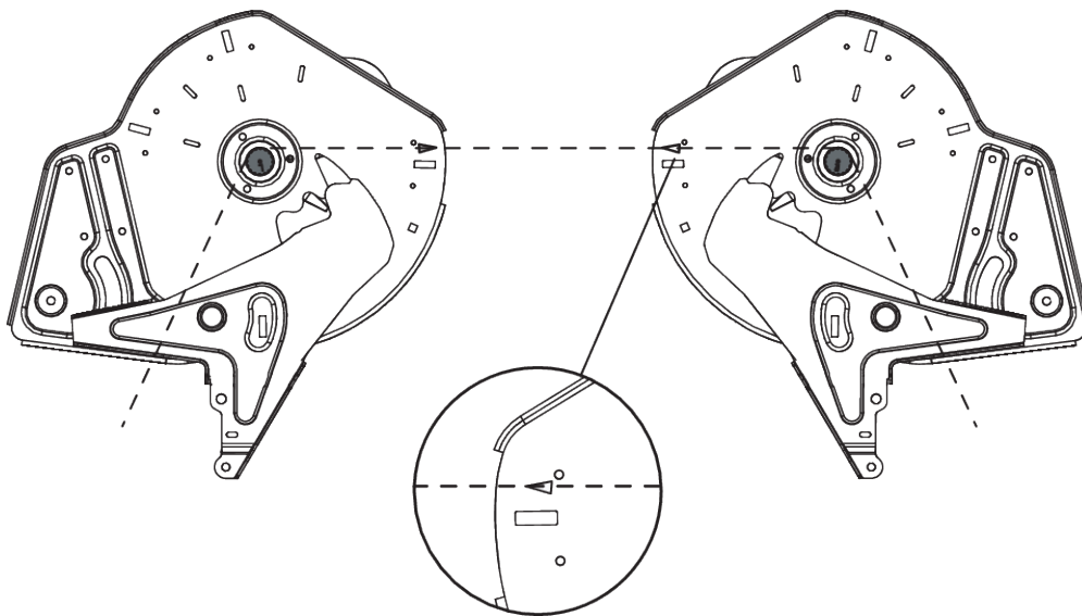
Pav. 63: Užduoties taško nustatymo patikra
