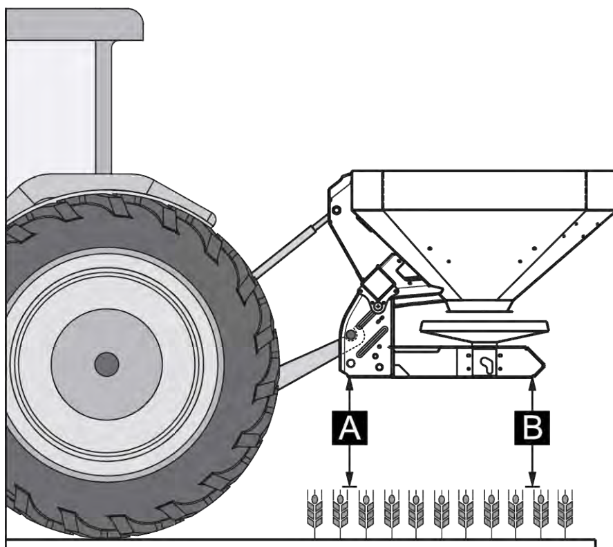
Pav. 19: Montavimo padėtis ir aukštis įprastajam tręšimui
