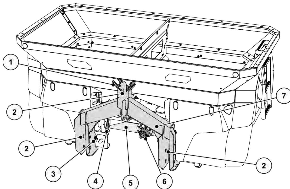
Pav. 6: Konstrukcinių grupių apžvalga: Priekinė pusė
