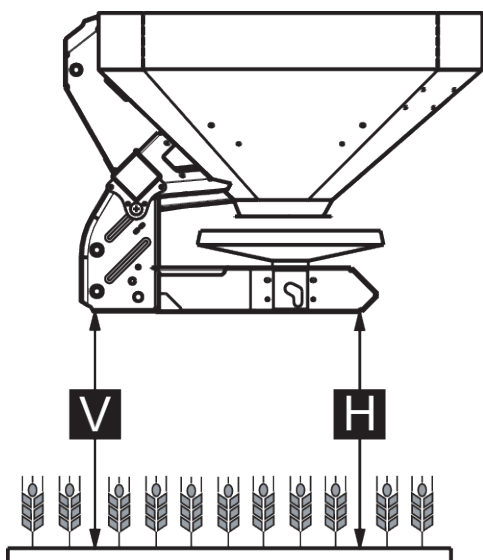
Pav. 18: Didžiausias leidžiamasis montavimo aukštis V ir H įprastajam ir vėlyvajam tręsimui
