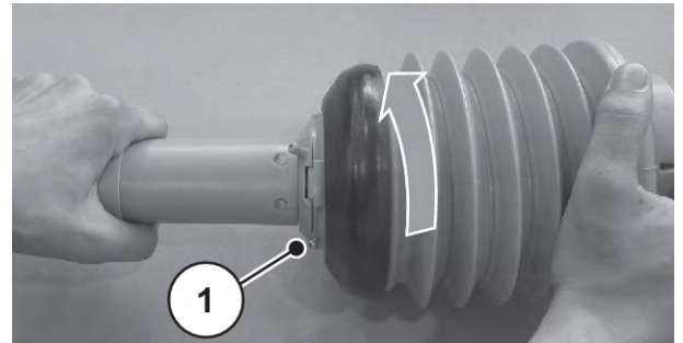
Pav. 10: Kardaninio veleno apsaugo atlaisvinimas
