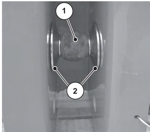
Pav. 16: Tarpinių diskų padėtis primontuojant mašiną
