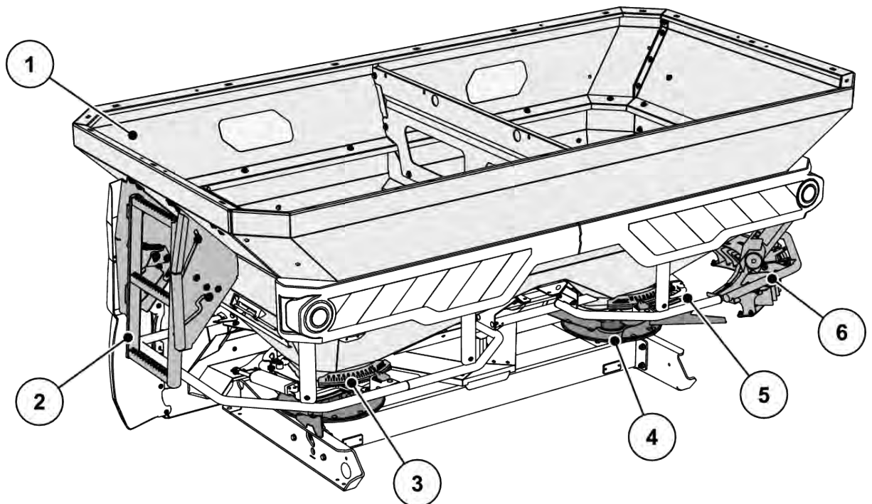
Pav. 5: Konstrukcinių grupių apžvalga: užpakalinė pusė
