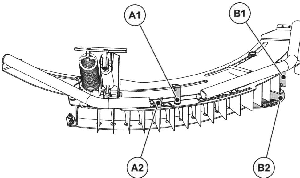
Pav. 23: TELIMAT Įrenginio nustatymas
