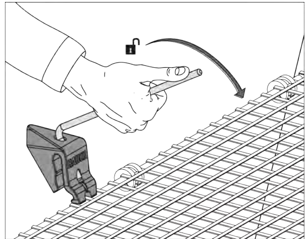
Pav. 50: Apsauginių grotelių fiksatoriaus atidarymas
