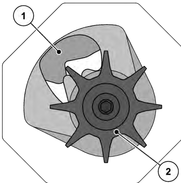
Jn. 8: Segamismehhanism
