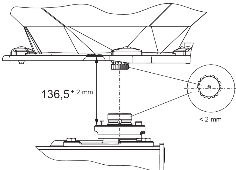
Ábr. 54: Szórótárcsaagy helyzetének ellenőrzése
