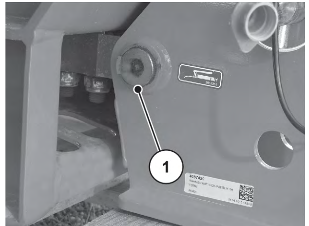
Ábr. 67: Mérleges műtrágyaszóró gép kenési pontja
