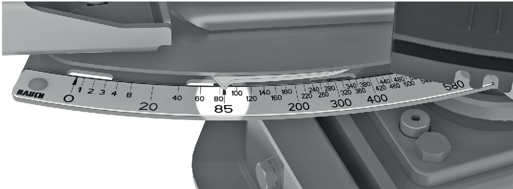
Ábr. 63: Adagoló tolóajtó mutatója a 85-ös skálaértéken
