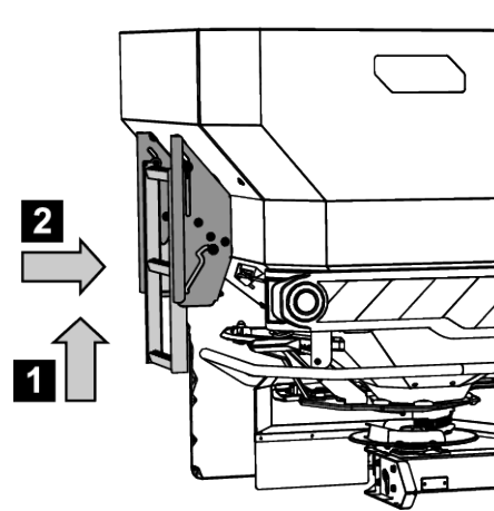
Ábr. 46: Fellépő behajtott állapotban
