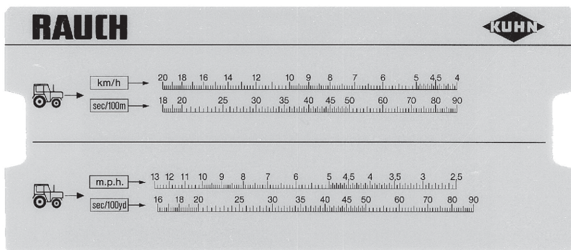
Ábr. 35: Skála a pontos menetsebesség megállapítására
