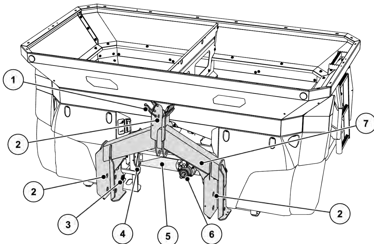
Ábr. 6: Részegységek áttekintése: első oldal
