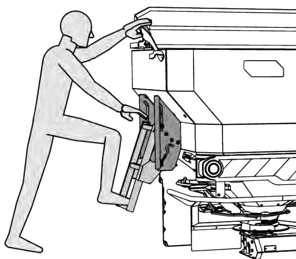
Ábr. 43: Létra tartály takaróponyvánal
