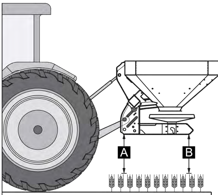
Ábr. 17: Felszerelési pozíció
