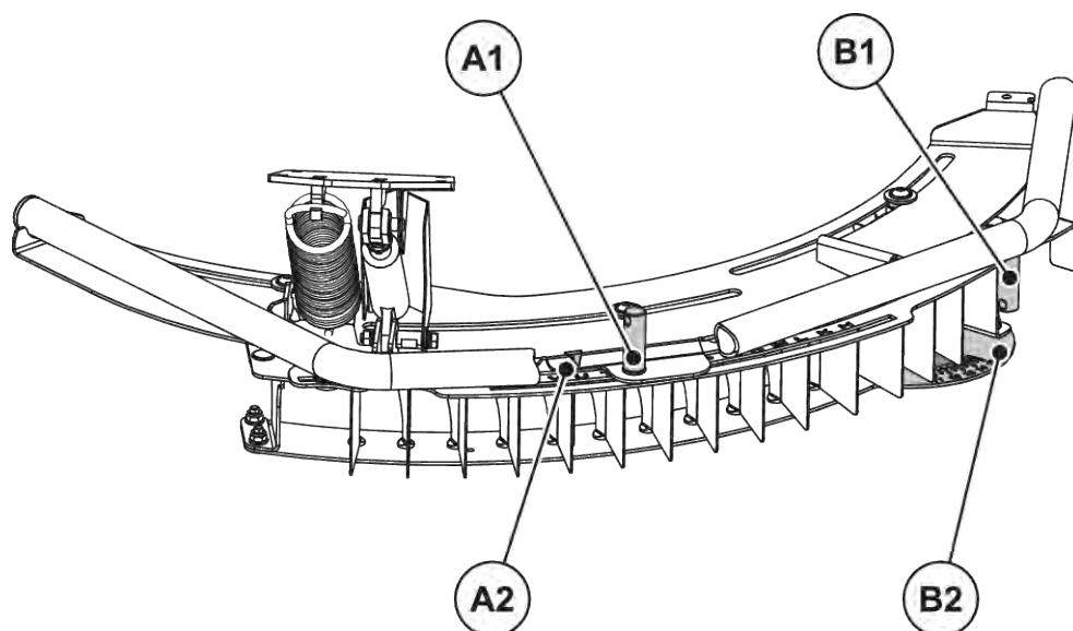
Ábr. 23: TELIMAT berendezés beállítása
