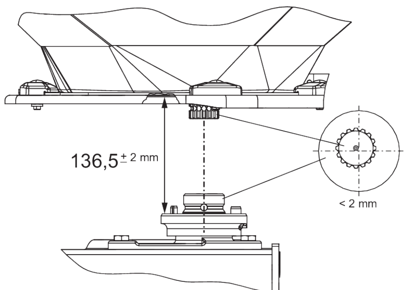
Sl. 53: Provera položaja glavčine diska za rasipanje
