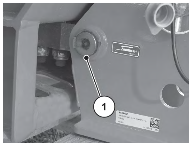
Sl. 66: Mesto podmazivanja mašine za rasipanje i vaganje
