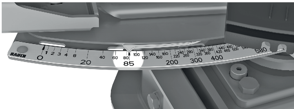
Sl. 62: Pokazivač klizača za doziranje na vrednosti 85 na skali
