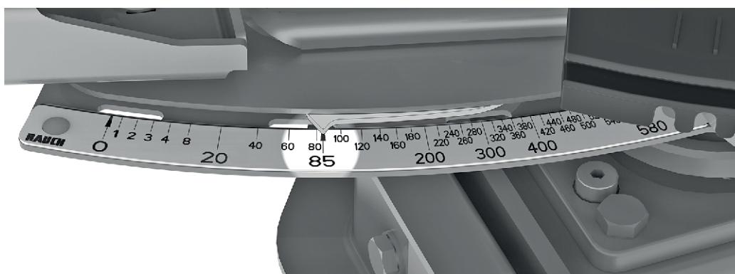
Рис. 62: Указатель заслонки дозатора на отметке 85
