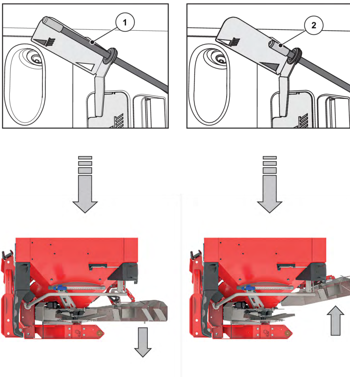
[1] GSE PRO разложен.
