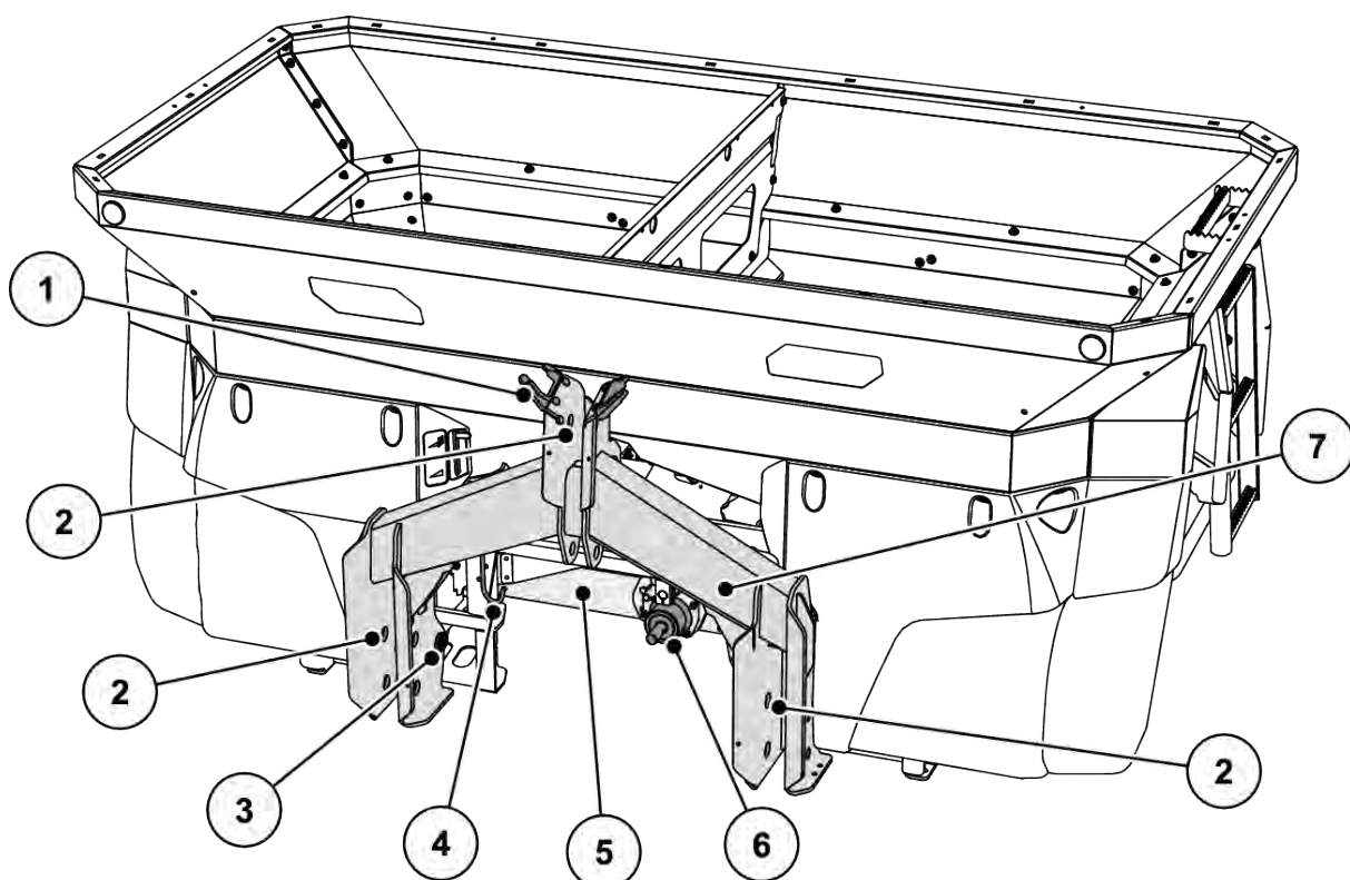
Рис. 6: Обзор конструктивных узлов: Передняя сторона
