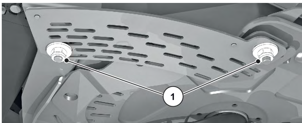
Рис. 61: Крепежные винты градуированной дуги
