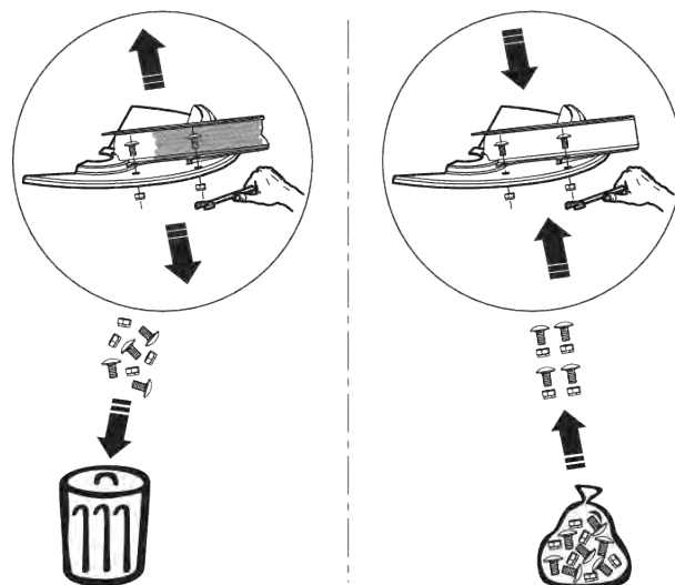
Рис. 58: Использование новых самоконтрящихся гаек
