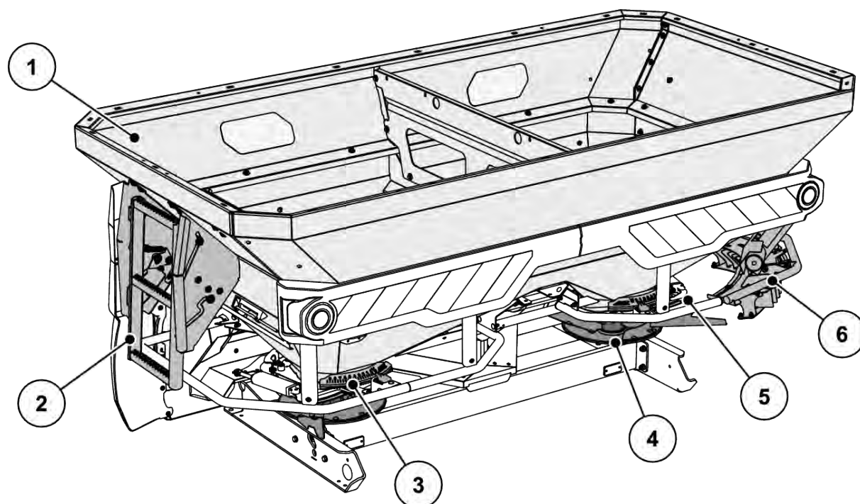
Рис. 5: Обзор конструктивных узлов: Задняя сторона
