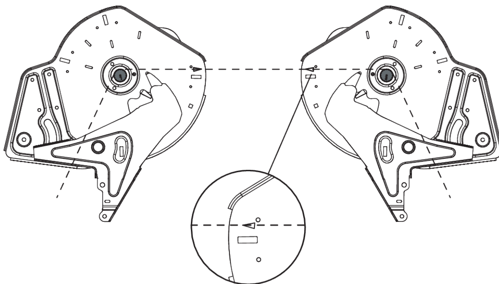
Рис. 63: Проверка настройки точки подачи
