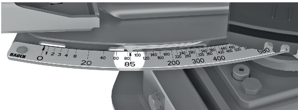
Fig. 62: Doseringsskyverpeker på skalaverdi 85
