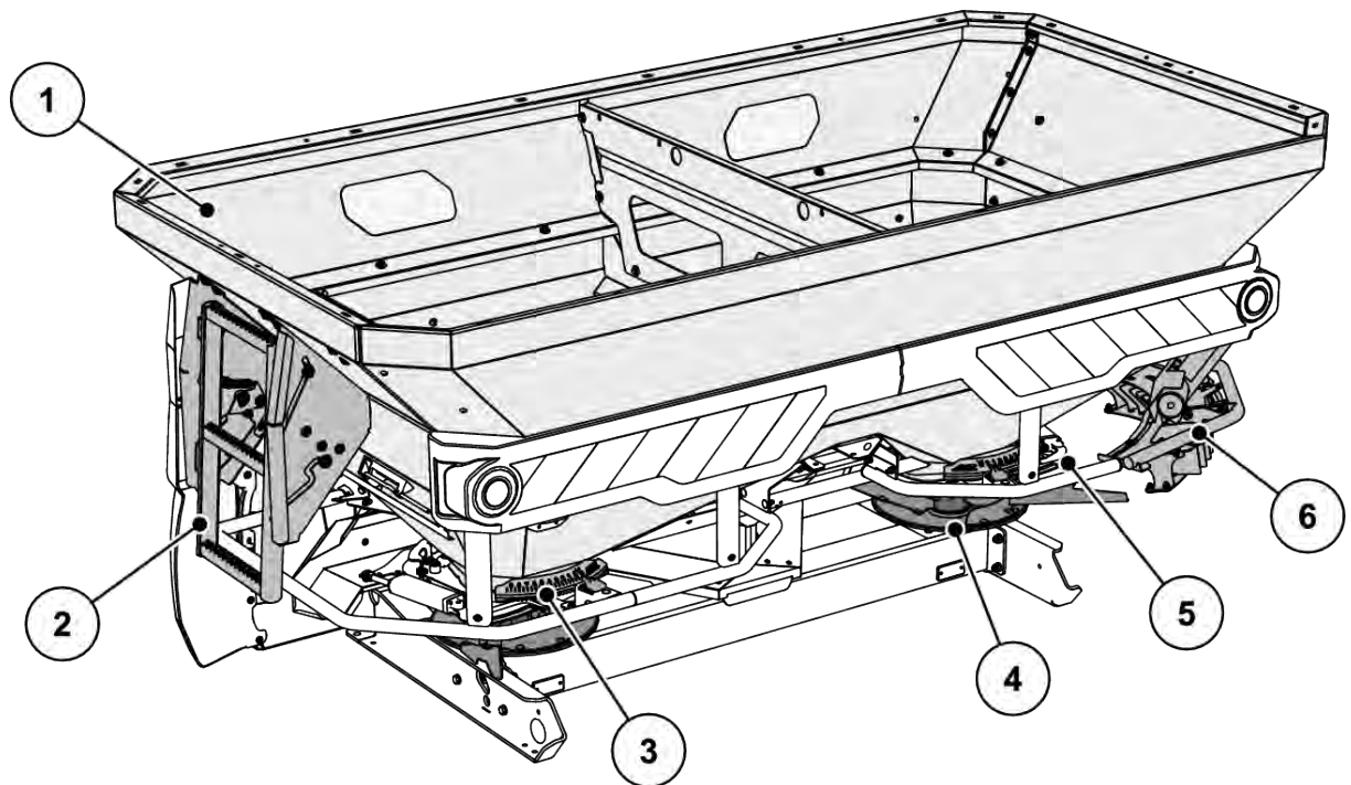
Fig. 5: Komponentoversikt: Bakside
