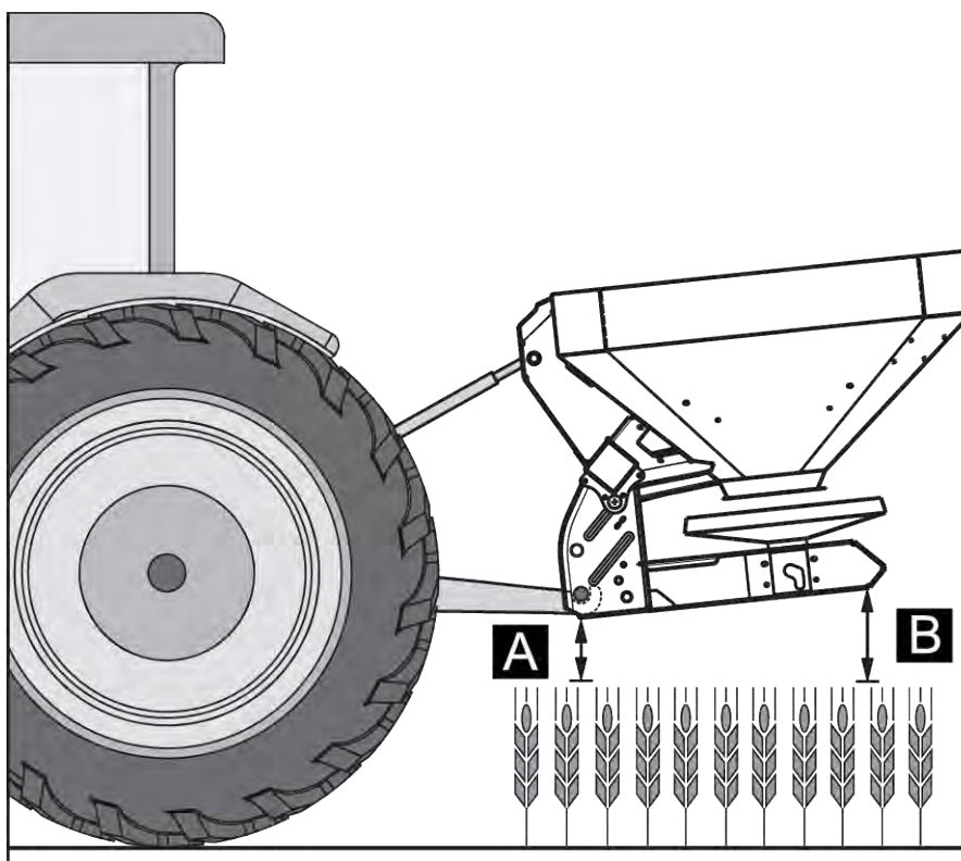
Fig. 21: Montering på maskinen på det nedre trekkstangkoblingspunktet
