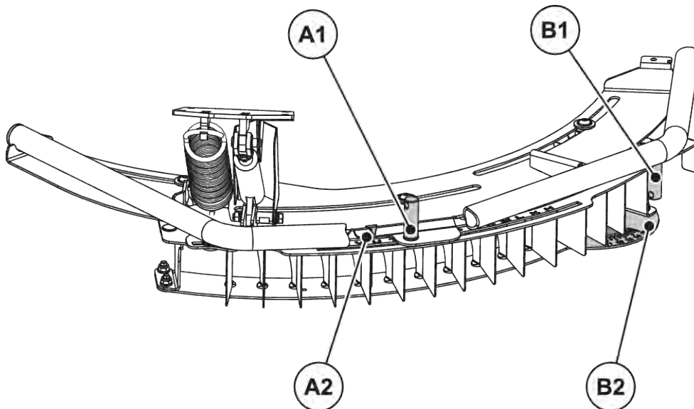
Obr. 24: Nastavení zařízení TELIMAT
