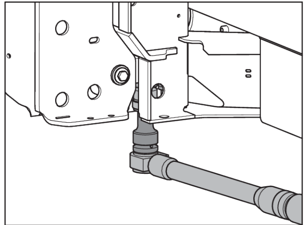
Obr. 47: Upevnění tenzometru (ve směru jízdy vlevo)
