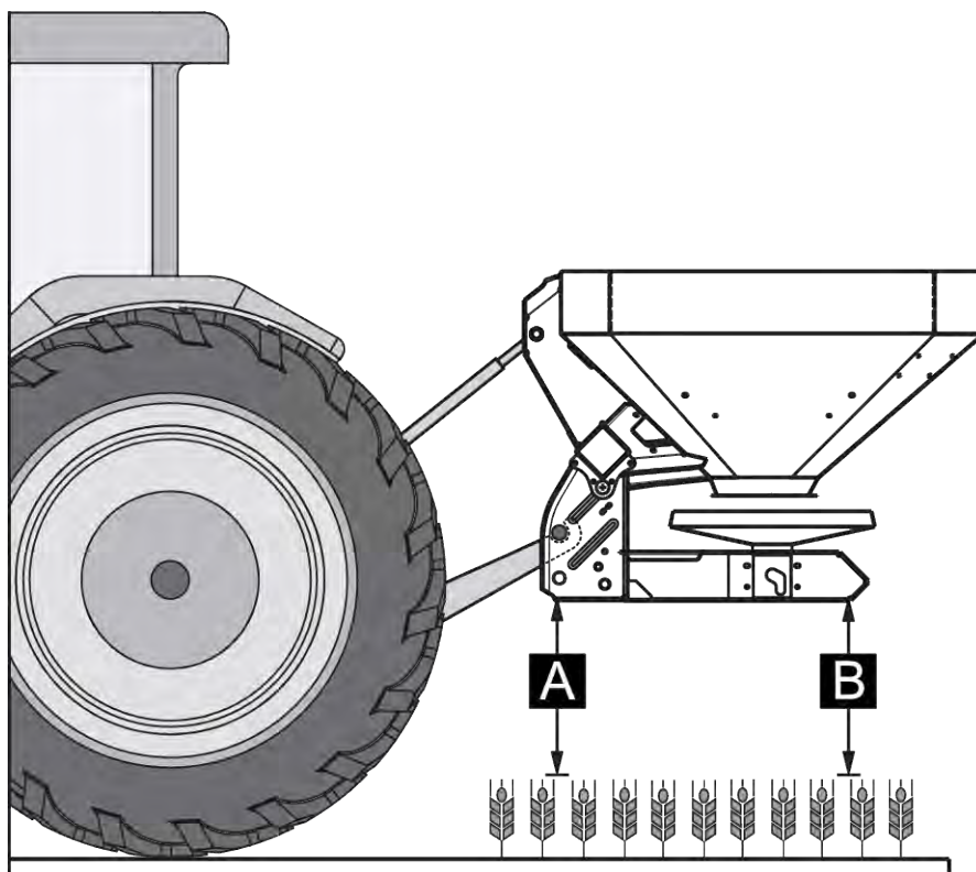
Obr. 17: Montážní poloha
