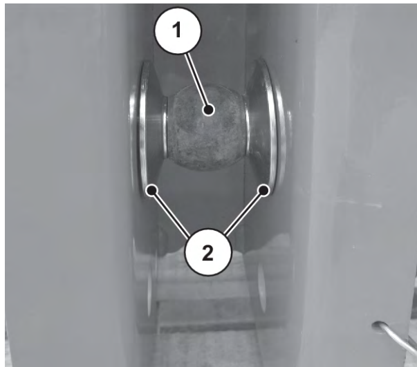
Obr. 16: Umístění vymezovacích podložek při montáži stroje
