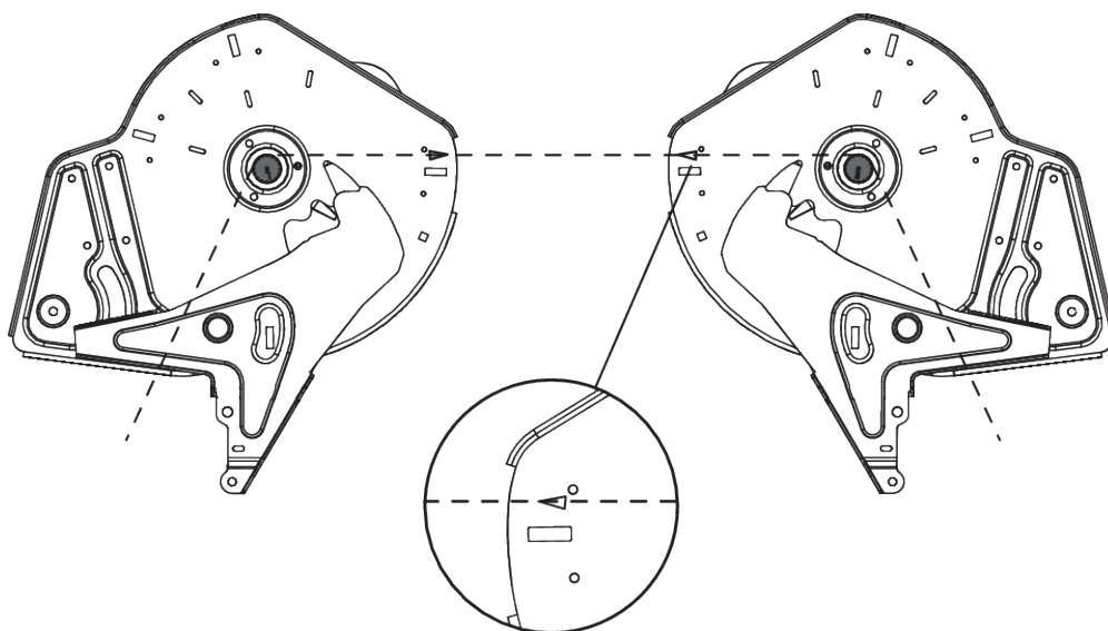
Obr. 63: Kontrola nastavení bodu výpadu
