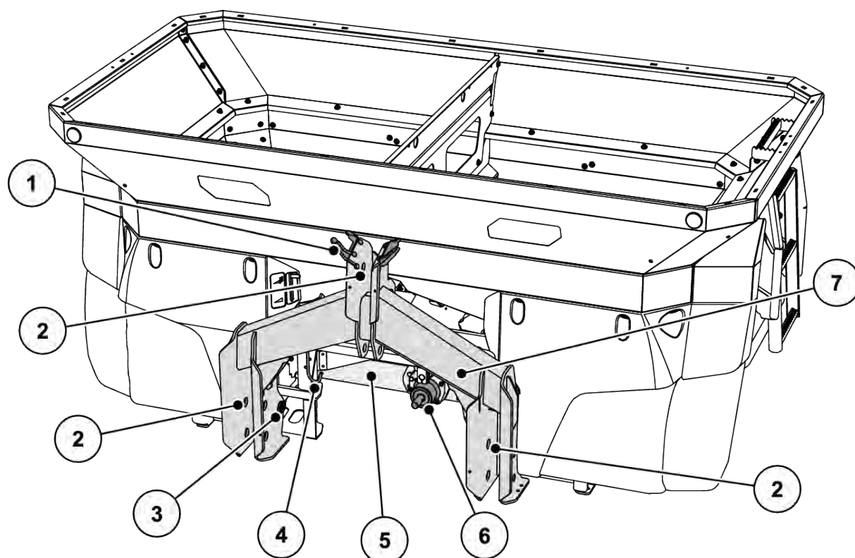
Obr. 6: Přehled konstrukčních skupin: Přední strana
