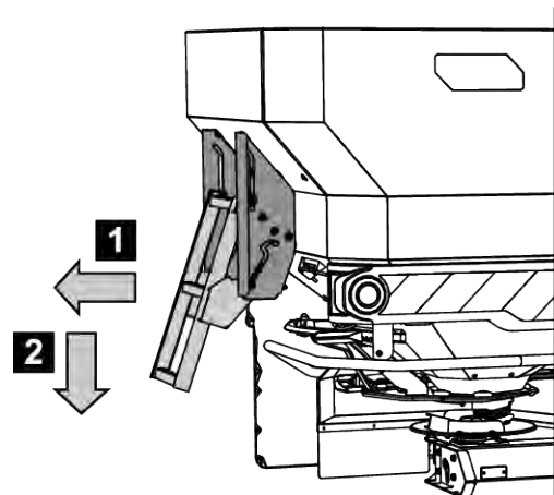
Fig. 45: Fälla ut fotsteg
