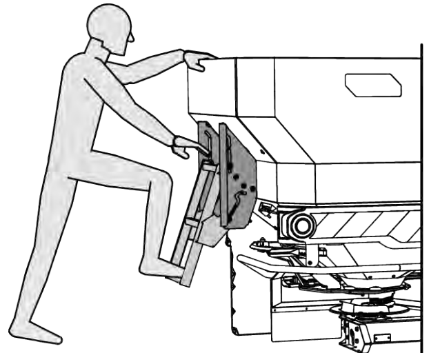
Fig. 43: Använda fotsteg utan behållarpresenning
