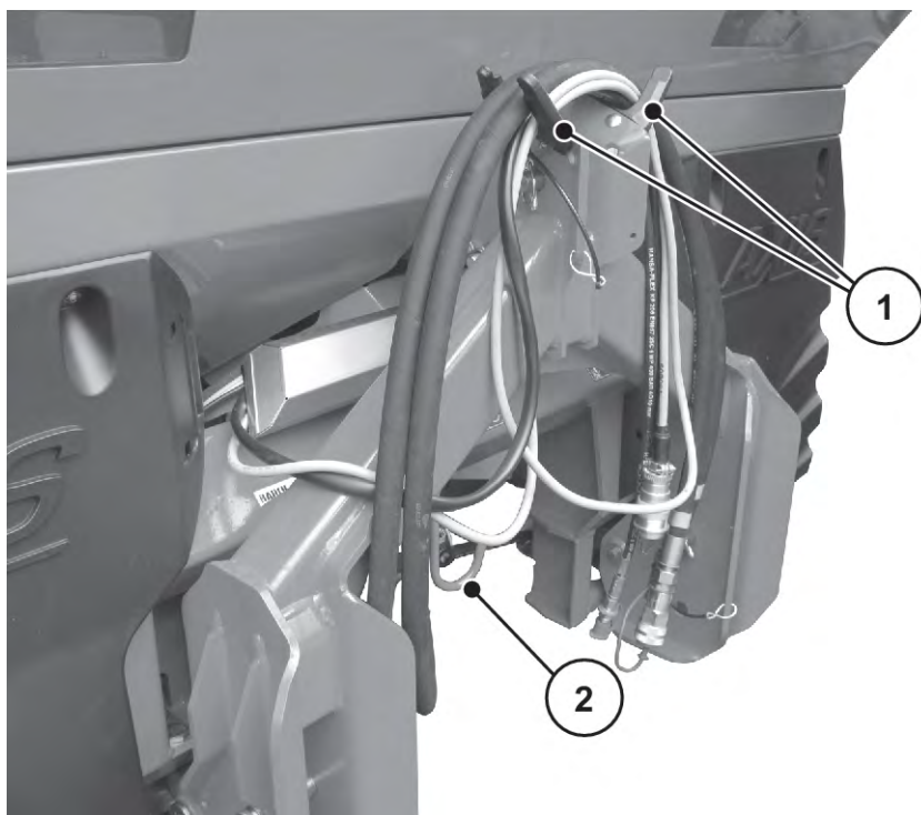
Fig. 42: Hållare för kablar och hydraulslangar
