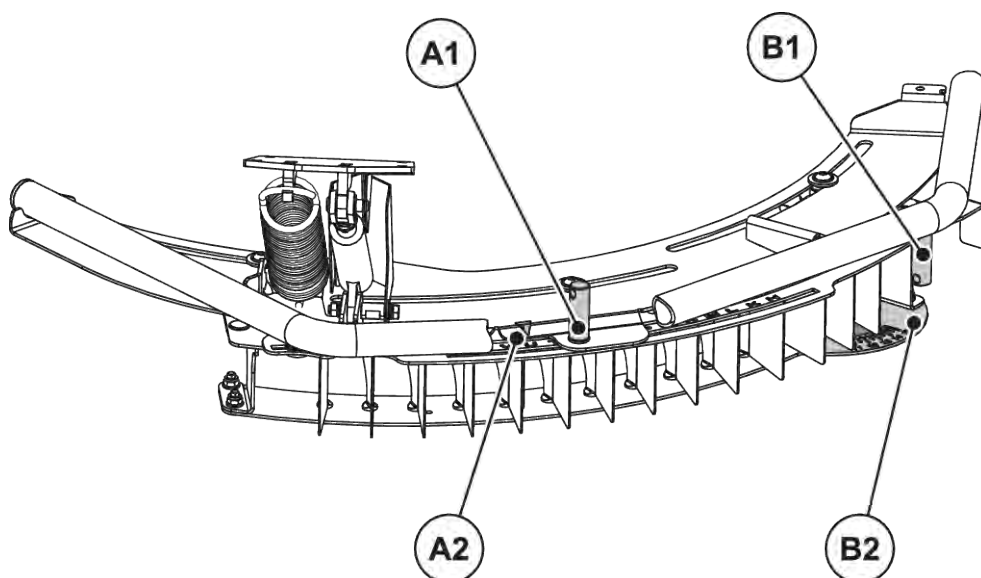
Fig. 24: Ställa in TELIMAT
