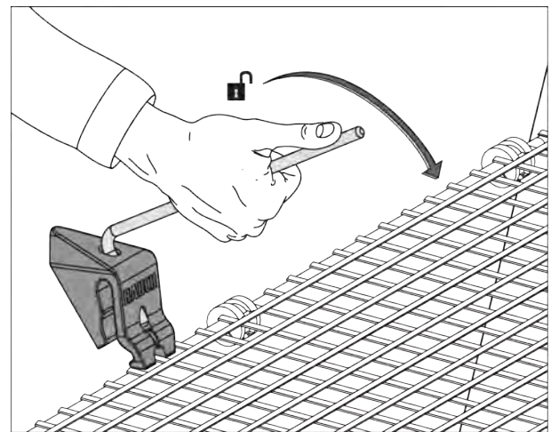
Fig. 51: Öppna skyddsgallerlåsningen
