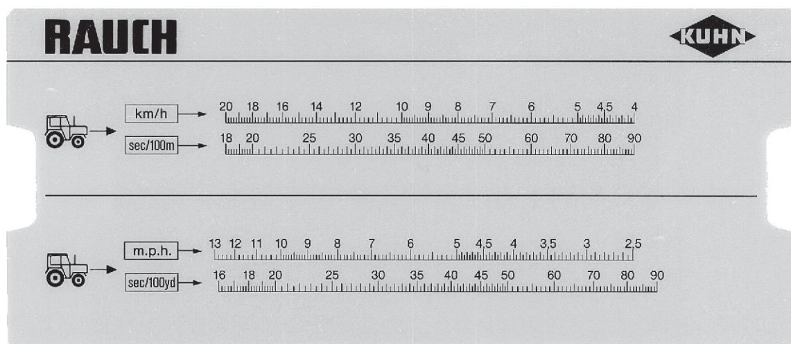
Fig. 35: Skala för beräkning av den exakta hastigheten
