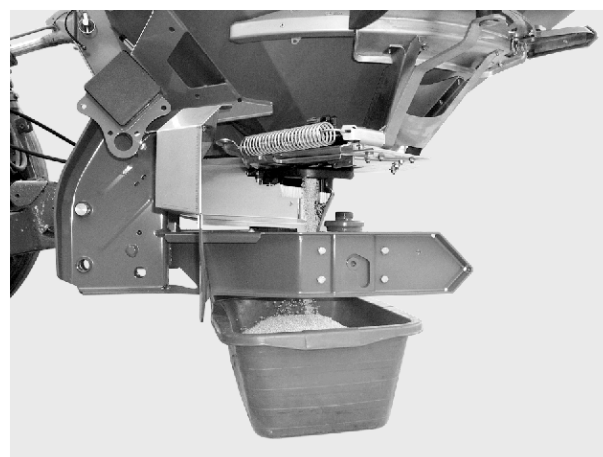
Fig. 40: Genomföra vridprov
