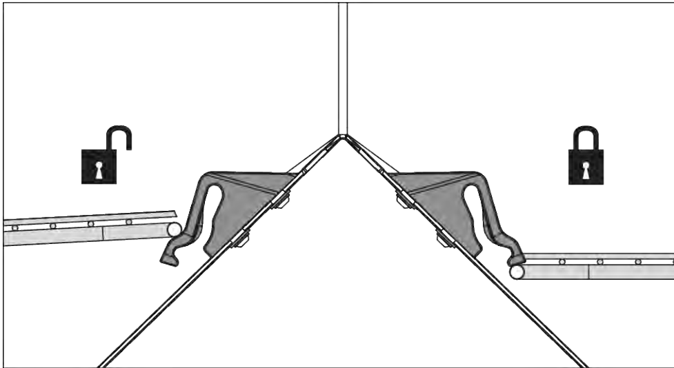
Fig. 50: Skyddsgallerlås öppet/stängt
