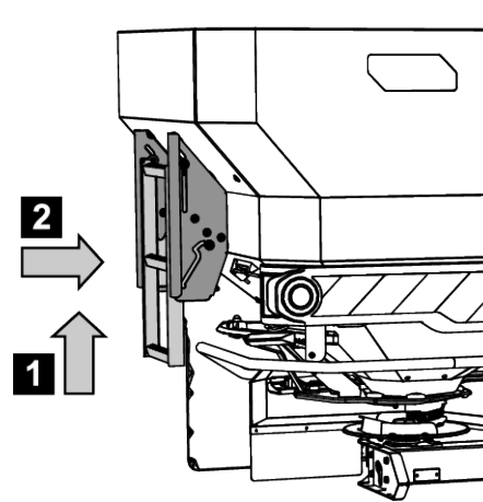
Fig. 46: Fotsteget i infällt läge.
