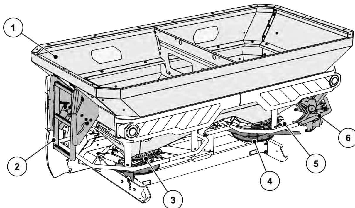
Fig. 5: Komponentgruppöversikt: Baksida
