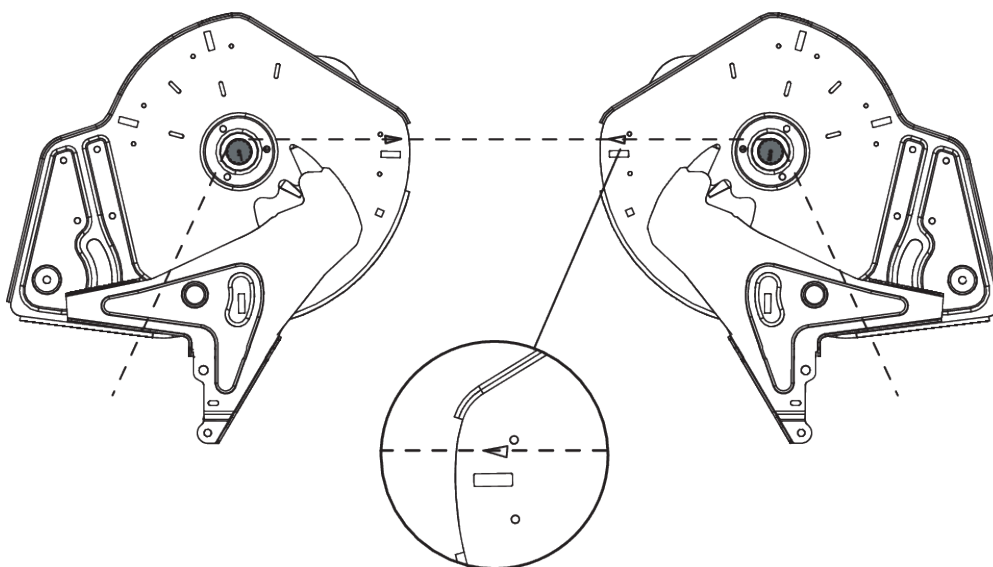
Fig. 63: Kontrollera inställningen av utmatningspunkten
