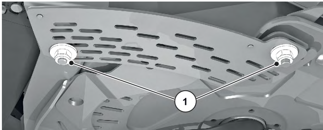
Fig. 61: Fästskruvar för skala
