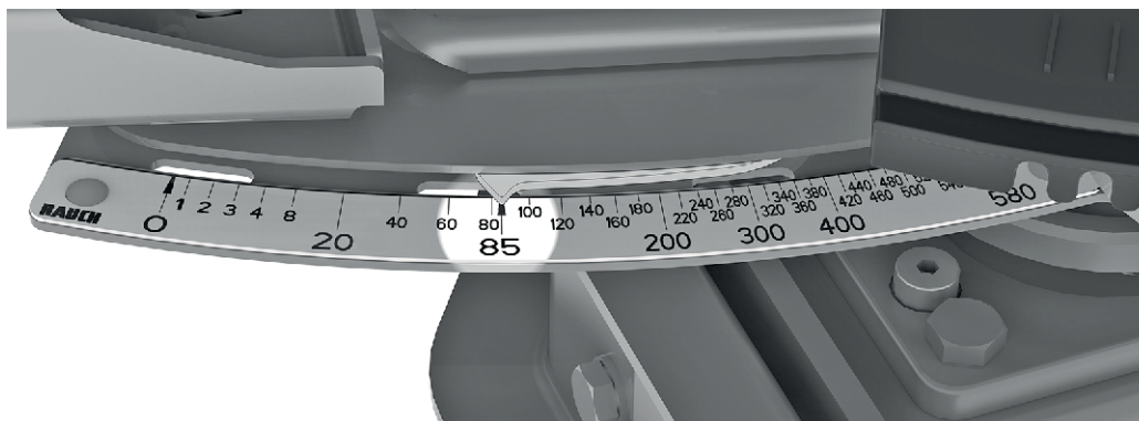
Fig. 62: Doseringsspjällets indikator visar på skalvärde 85.
