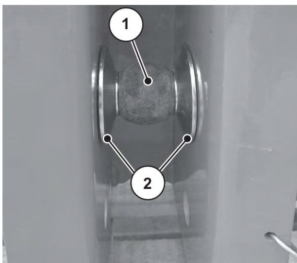
Fig. 16: Distansbrickornas läge vid montering av maskinen
