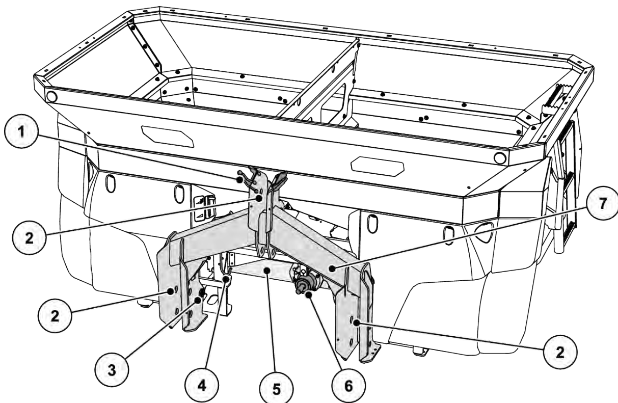
Fig. 7: Moduloversigt: Forside
