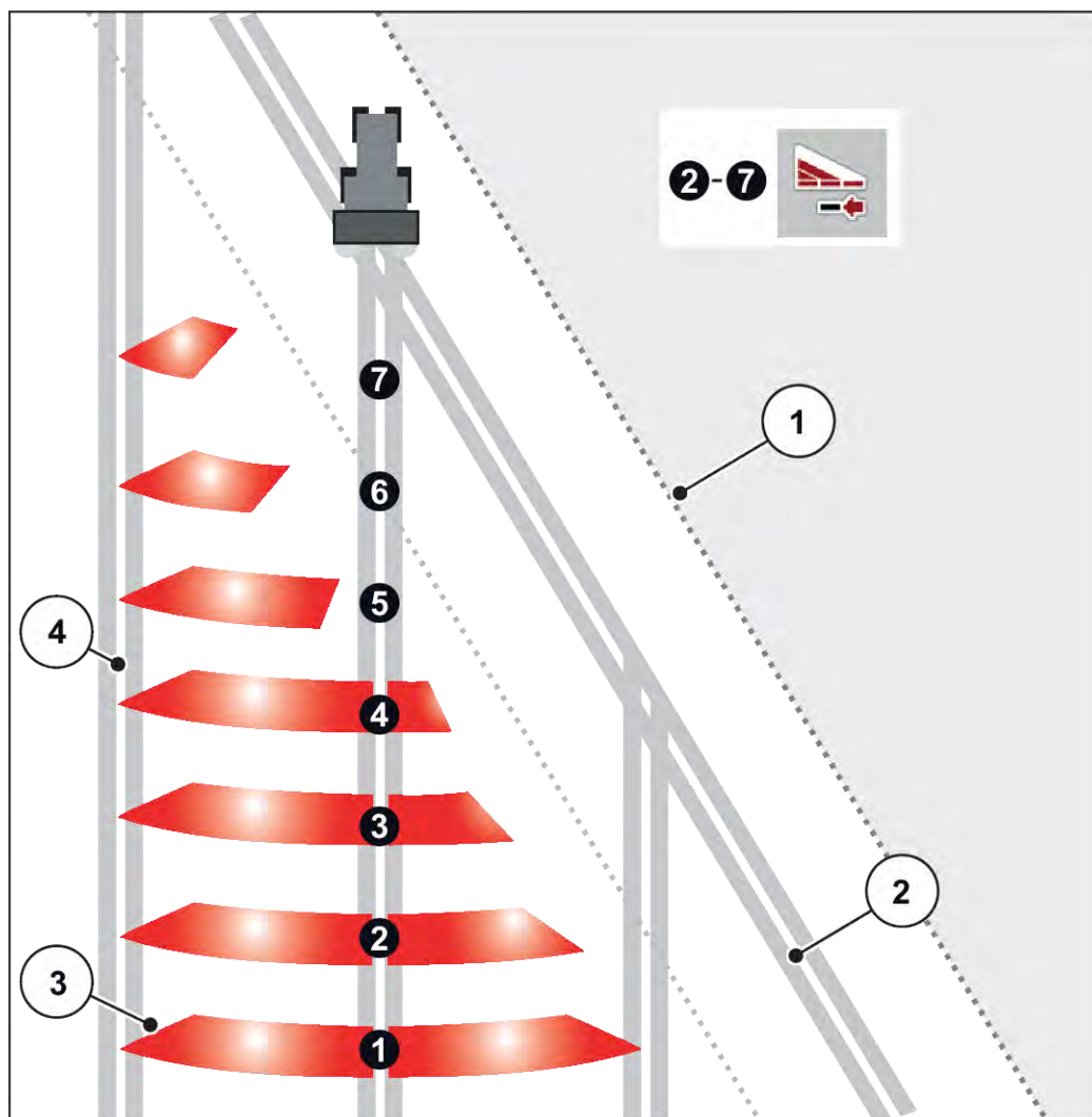
Fig. 34: Eksempel på delbreddekobling med VariSpread pro
