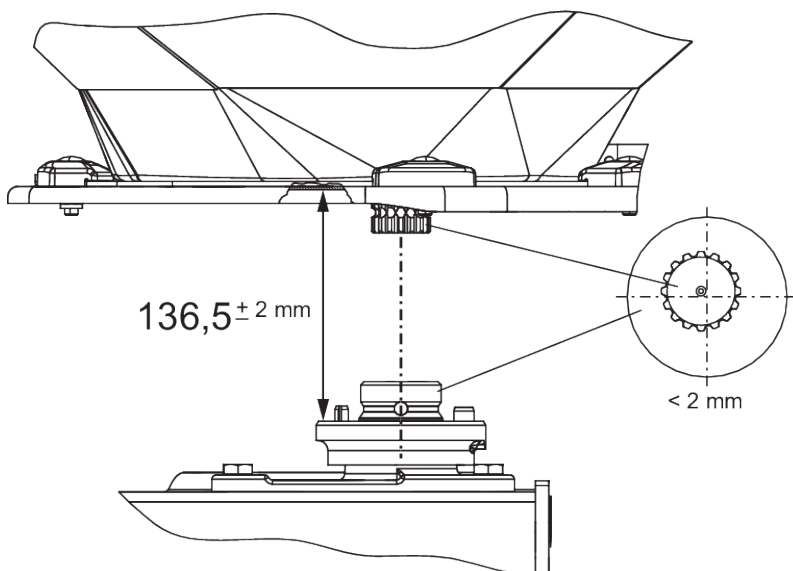
Fig. 54: Kontrol af position for spredskivenav
