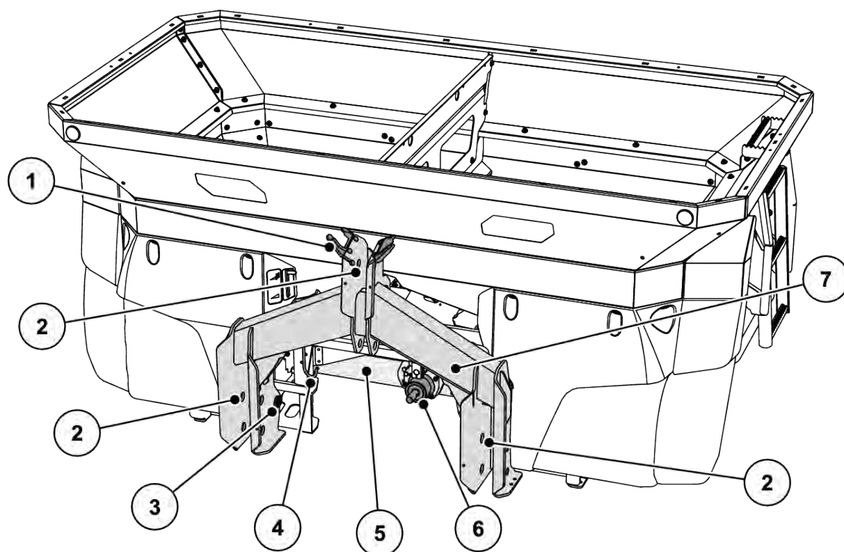
Fig. 6: Moduloversigt: Forside
