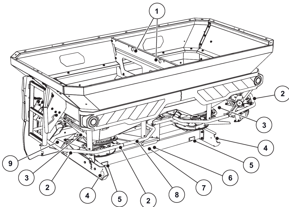
Fig. 3: Beskyttelsesordninger samt advarsels- og instruktionsmærkater på bagsiden
