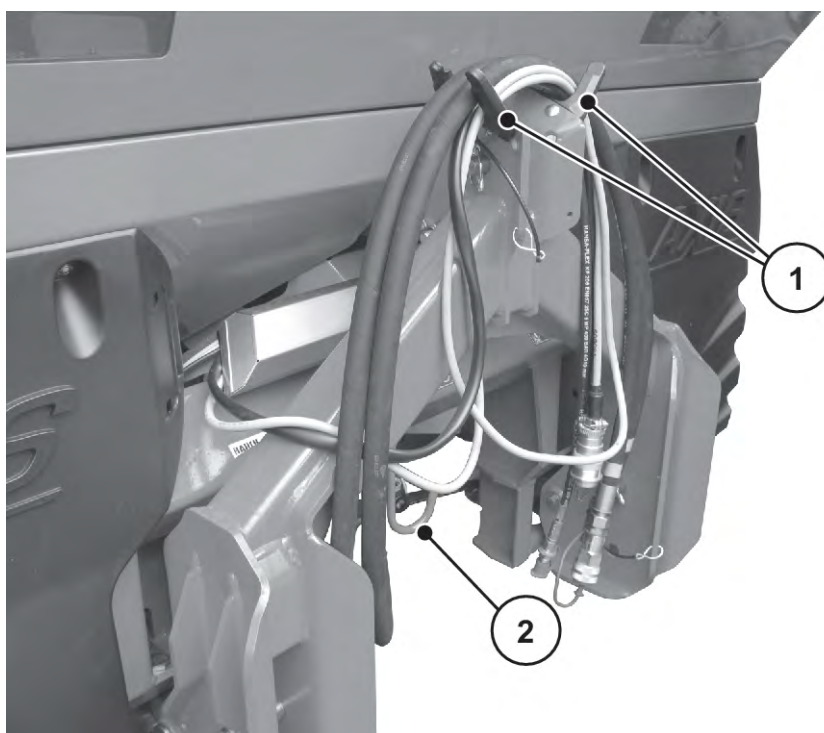
Fig. 15: Holder til kabler og hydraulikslanger
