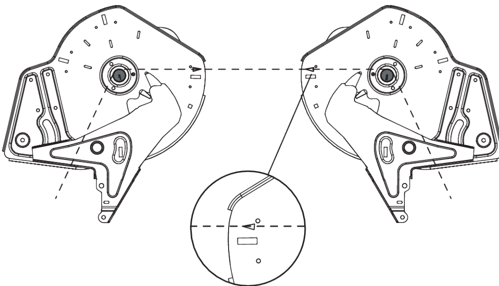
Fig. 63: Kontrol af indstillingen af udbringningspunktet
