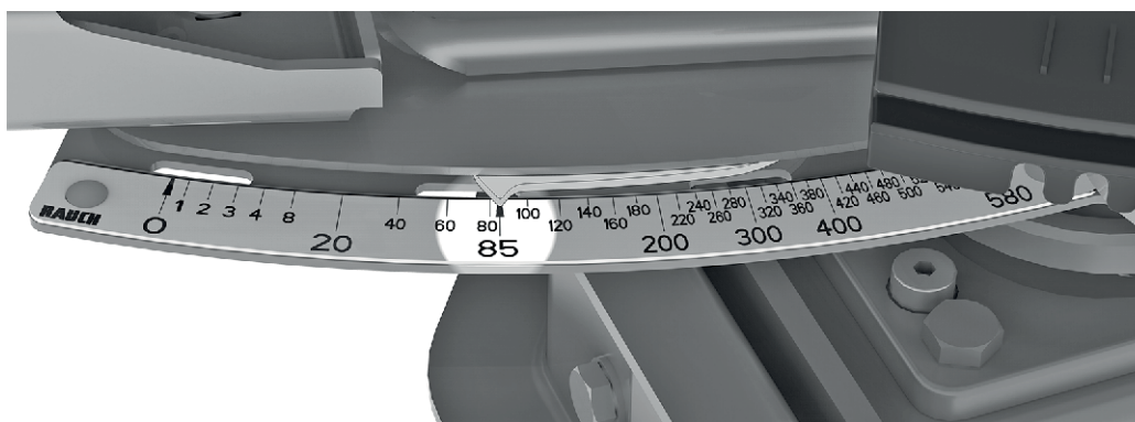
Fig. 62: Doseringsspjældviser på skalaværdi 85
