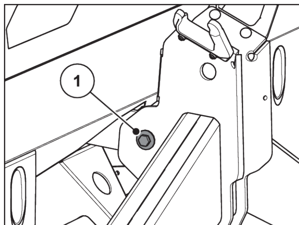
Fig. 47: Fastgørelse af trækstaven på vejerrammen
