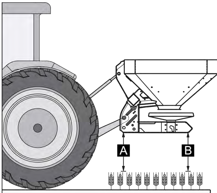
Fig. 19: Monteringsposition og -højde ved normal gødning
