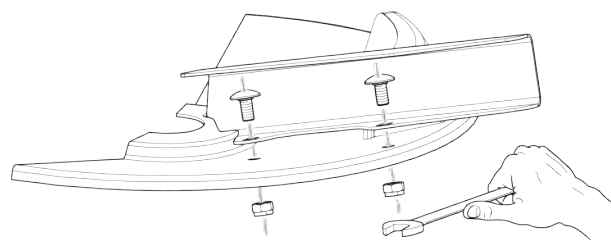
Fig. 57: Løsning af skruerne på spredvingen
