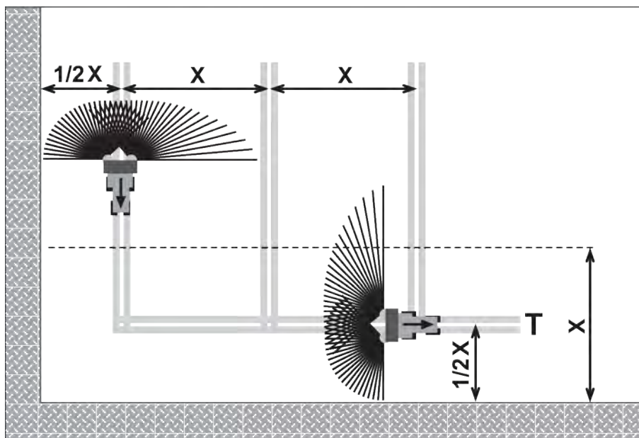
Afb. 31: Grensstrooien
