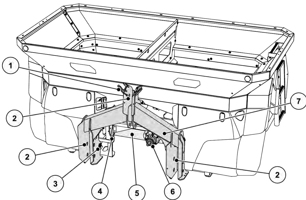
Afb. 6: Module-overzicht: Voorzijde
