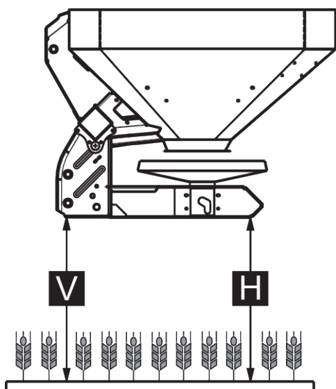
Afb. 18: Maximaal toegestane aanbouwhoogte in de normale en late bemesting
