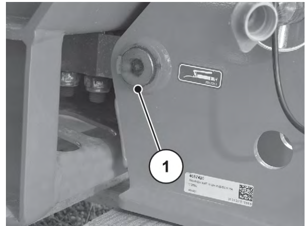
Fig. 66: Punct de lubrifiere la distribuitorul cu cântărire
