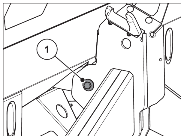
Fig. 47: Fixarea tijei de tracțiune pe cadrul de cântărire
