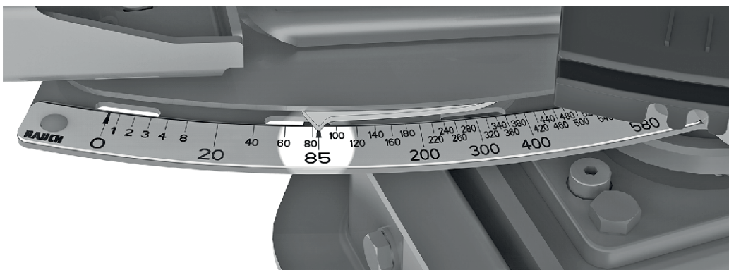
Σχ. 62: Δείκτης συρόμενου δοσομετρητή στην τιμή κλίμακας 85
