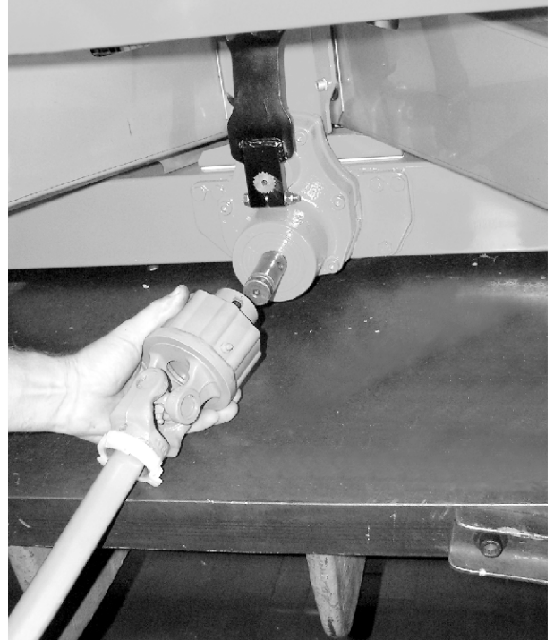
Σχ. 11: Πέρασμα αρθρωτού άξονα σε στροφέα κιβωτίου μετάδοσης
