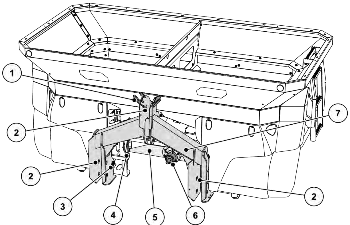
Σχ. 6: Επισκόπηση κατασκευαστικών ομάδων: Μπροστινή πλευρά
