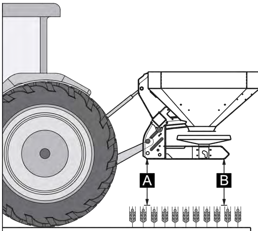
Σχ. 17: Θέση προσάρτησης
