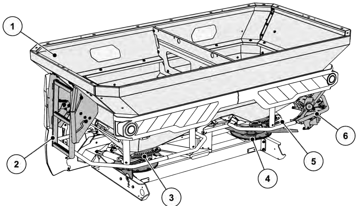
Σχ. 5: Επισκόπηση κατασκευαστικών ομάδων: Πίσω πλευρά
