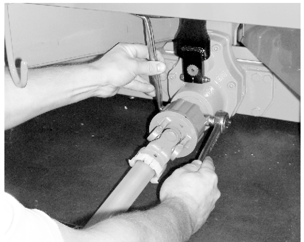
Σχ. 12: Στερέωση αρθρωτού άξονα
