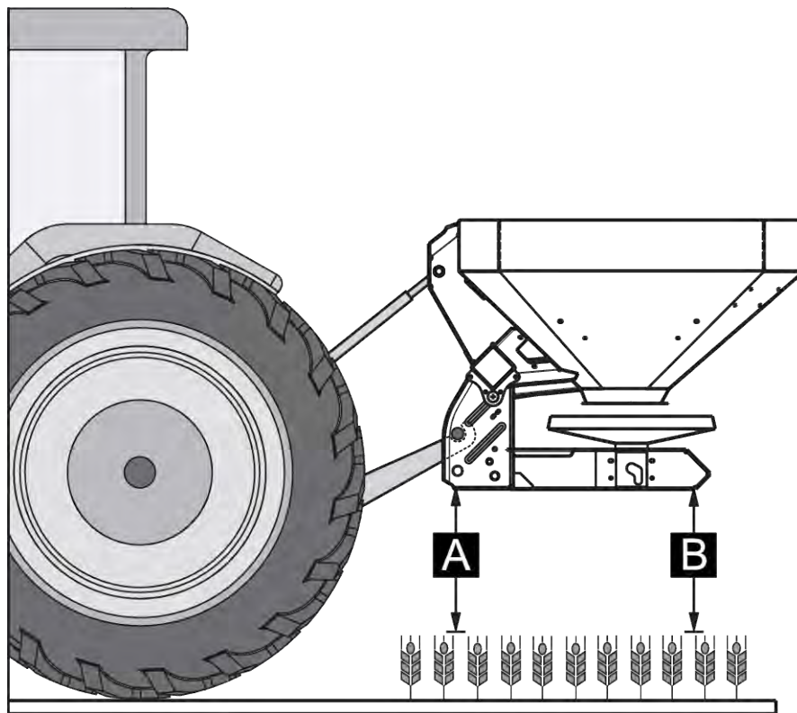
Σχ. 19: Θέση και ύψος προσάρτησης στην κανονική λίπανση
