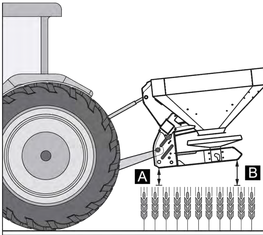
Σχ. 20: Θέση και ύψος προσάρτησης στην όψιμη λίπανση
