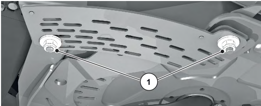
Σχ. 61: Βίδες στερέωσης της κλίμακας
