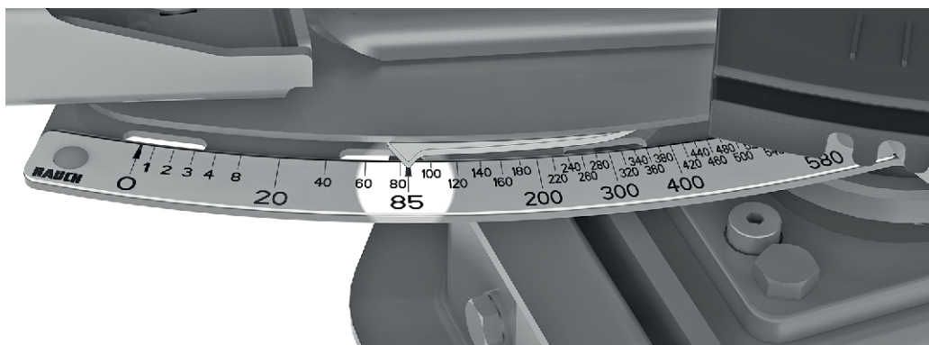
Фиг. 62: Стрелка на дозиращия шибър до стойност на скалата 85
