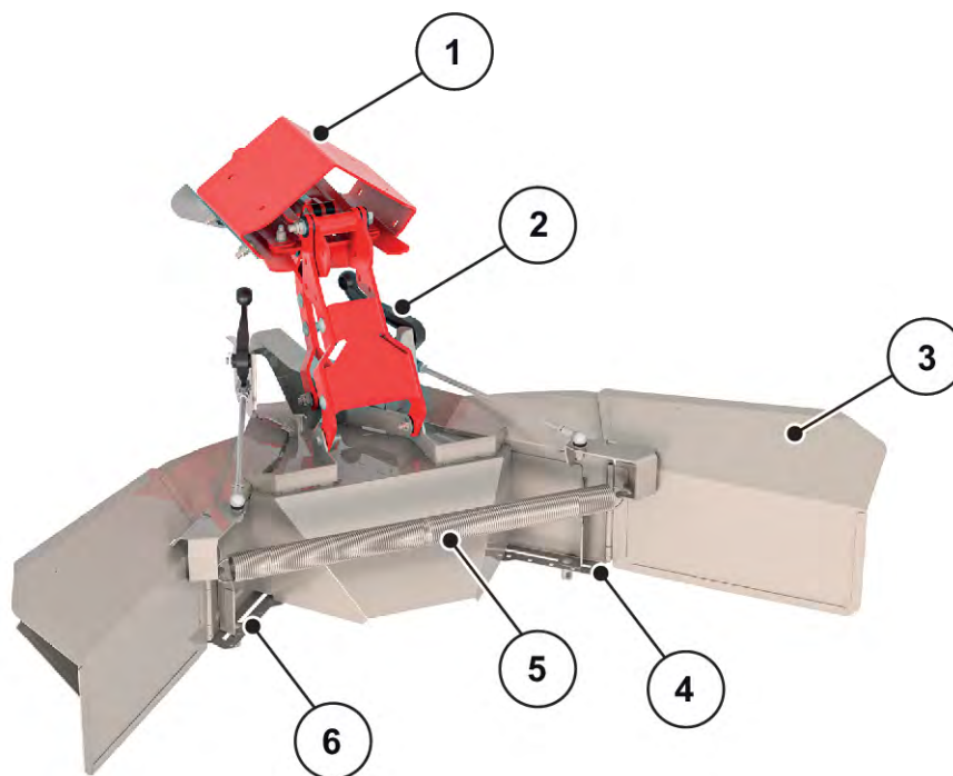
Фиг. 22: Настройване на устройството за гранично разпръскване
