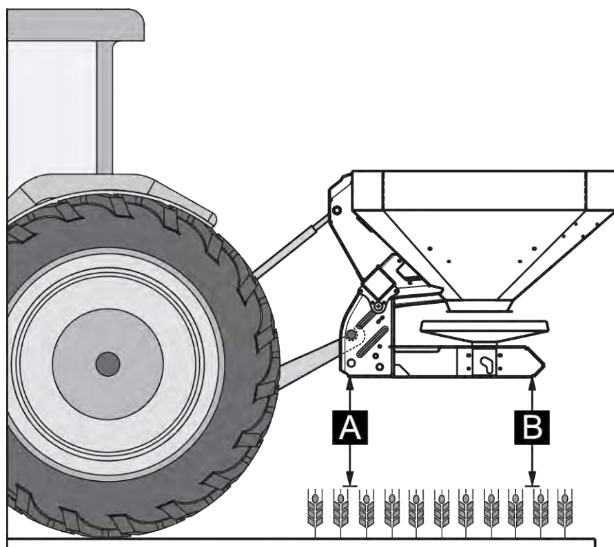
Фиг. 17: Позиция за прикачване
