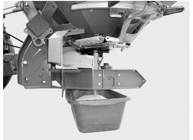
Rys. 40: Wykonanie próby rozsiewu
