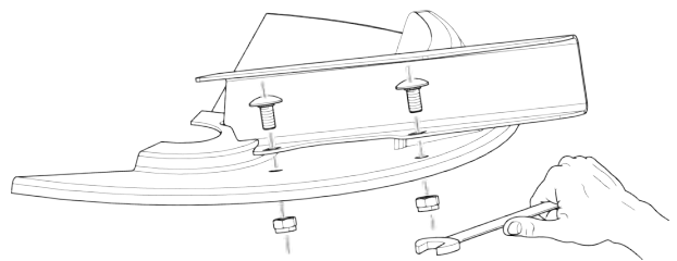
Rys. 58: Odkręcanie śrub łopatek rozrzucających
