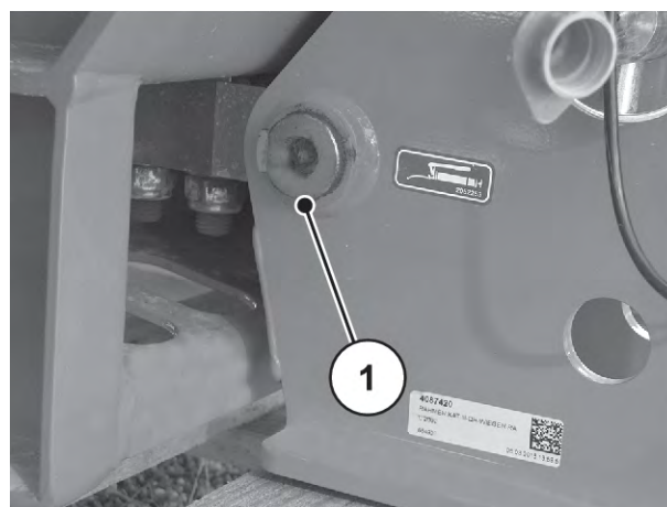
Rys. 67: Punkt smarowania rozsiewacza wagowego
