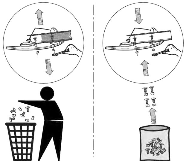
Rys. 59: Używać nowych nakrętek samozabezpieczających
