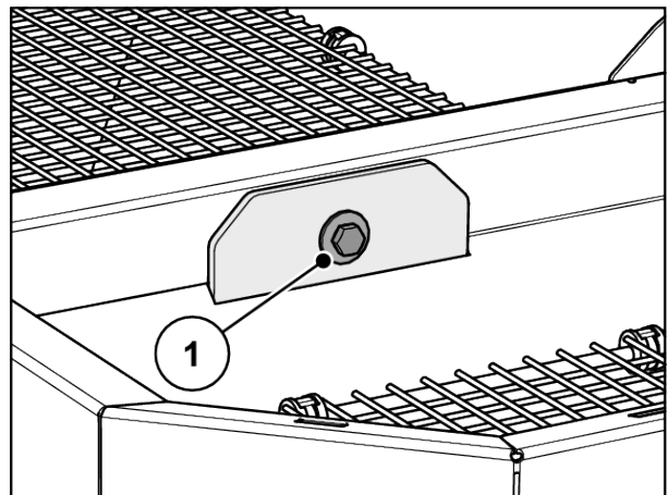
Rys. 49: Mocowanie cięgła w zbiorniku
