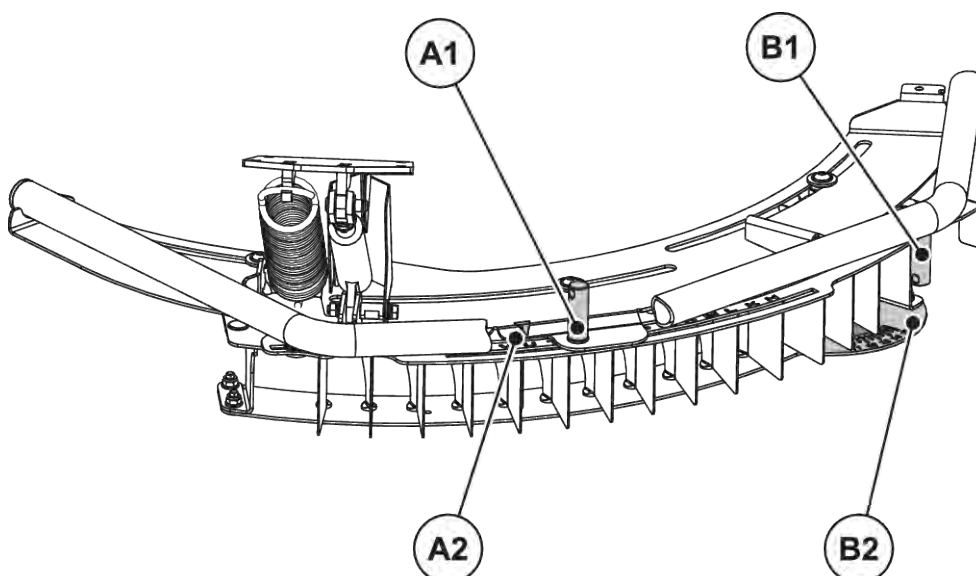
Rys. 23: Ustawianie urządzenia TELIMAT
