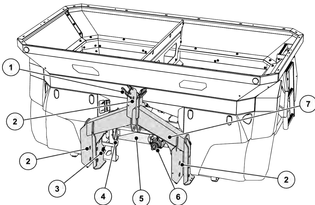
Rys. 6: Widok ogólny zespołów: Widok od przodu
